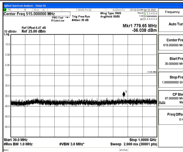
Band4-5MHz-QPSK-20175-1-0-Low-30-1000--36.04-PASS
