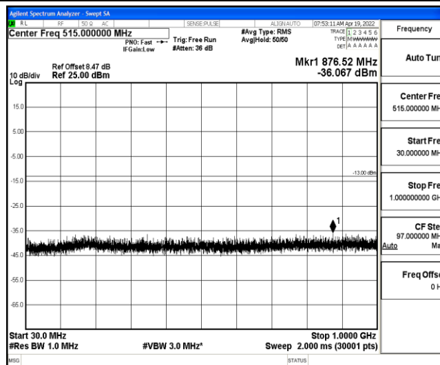
Band4-10MHz-QPSK-20175-1-0-Low-30-1000--36.07-PASS
