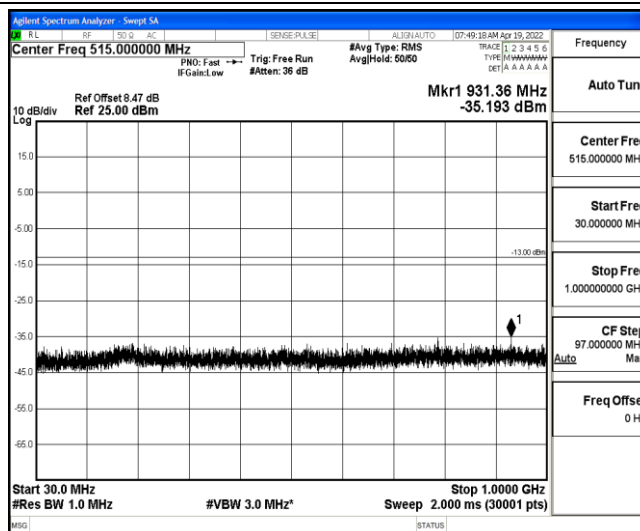
Band4-10MHz-QPSK-20000-1-0-Low-30-1000--35.19-PASS
