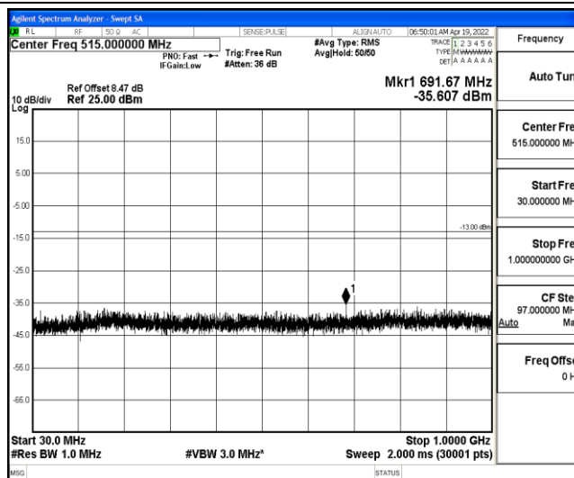
Band4-3MHz-QPSK-19965-1-0-Low-30-1000--35.61-PASS
