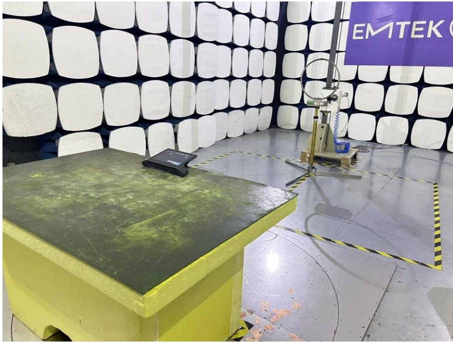
Test Setup (Below 30MHz)
