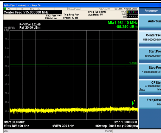
Band2-20MHz-QPSK-19100-1-0-Low-30-1000--59.24-PASS
