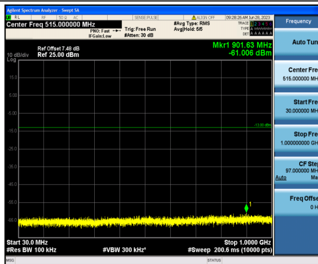
Band4-5MHz-QPSK-20375-1-0-Low-30-1000--61.01-PASS
