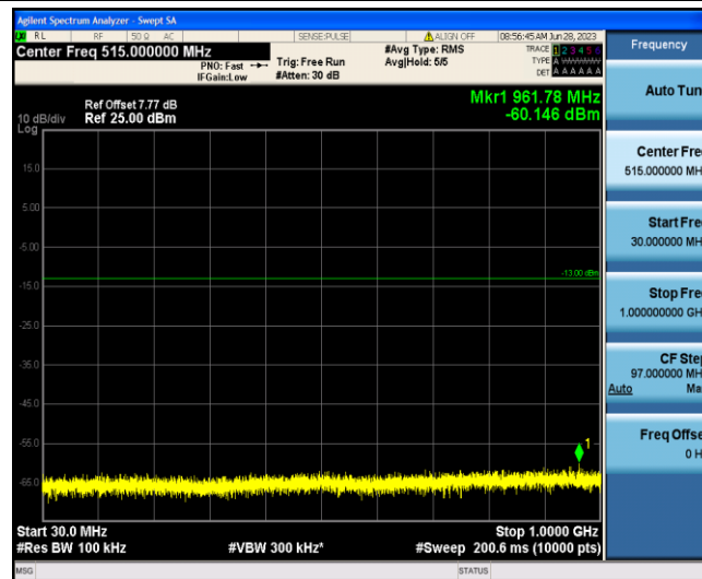
Band4-1.4MHz-QPSK-19957-1-0-Low-30-1000--60.15-PASS
