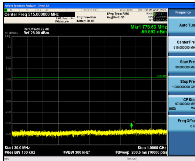
Band2-20MHz-QPSK-18700-1-0-Low-30-1000--59.59-PASS
