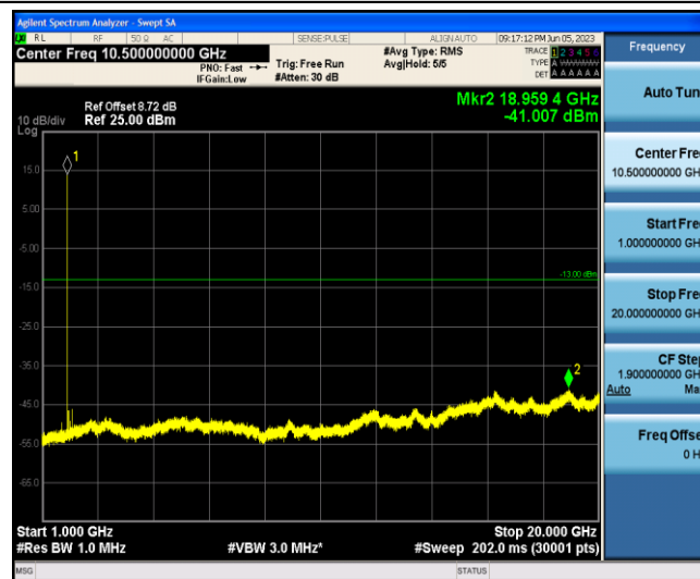
Band2-20MHz-16QAM-18700-1-0-Low-1000-20000--41.01-PASS
