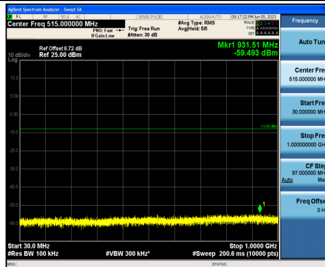
Band2-20MHz-QPSK-18900-1-0-Low-30-1000--59.49-PASS
