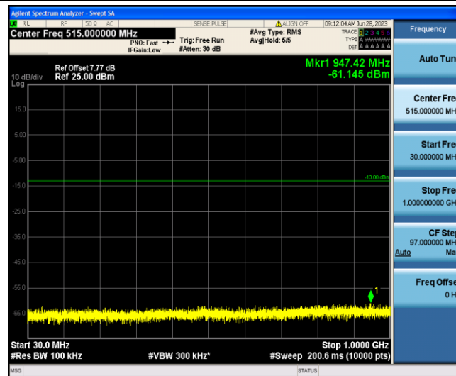
Band4-3MHz-QPSK-19965-1-0-Low-30-1000--61.15-PASS
