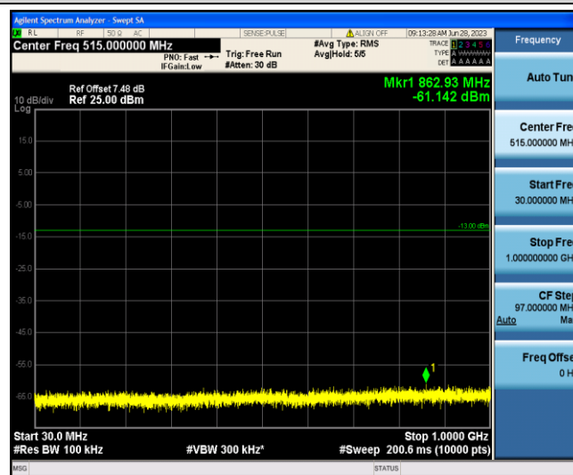
Band4-3MHz-QPSK-20385-1-0-Low-30-1000--61.14-PASS
