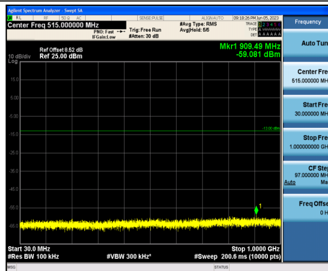
Band2-20MHz-16QAM-19100-1-0-Low-30-1000--59.08-PASS
