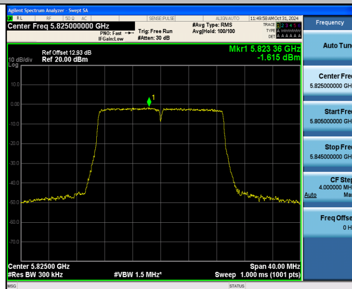
11AC20MIMO_Ant2_5825
