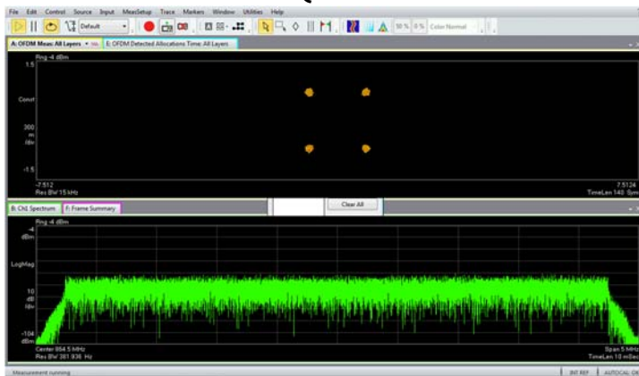
QPSK
