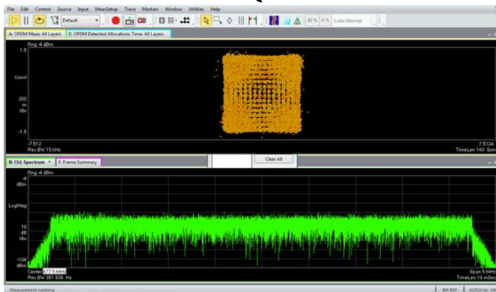
256QAM
