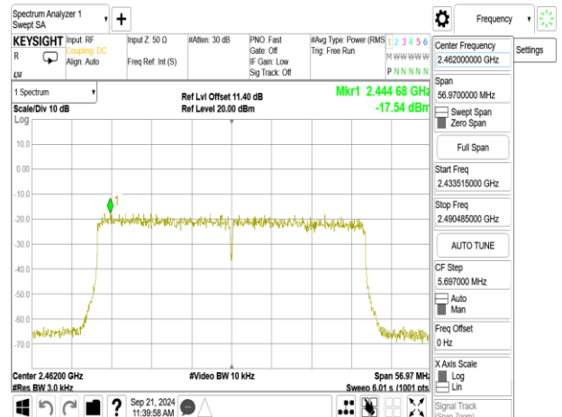
802.11be_40MHz_ChainB_2462MHz_RU242_62
