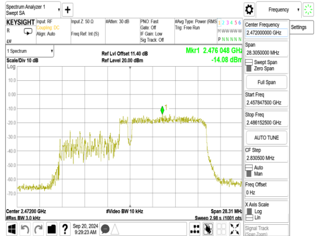
802.11be_20MHz_ChainB_2472MHz_52+26_MR03
