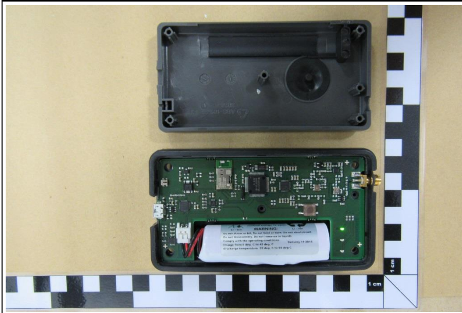
EUT OPEN
