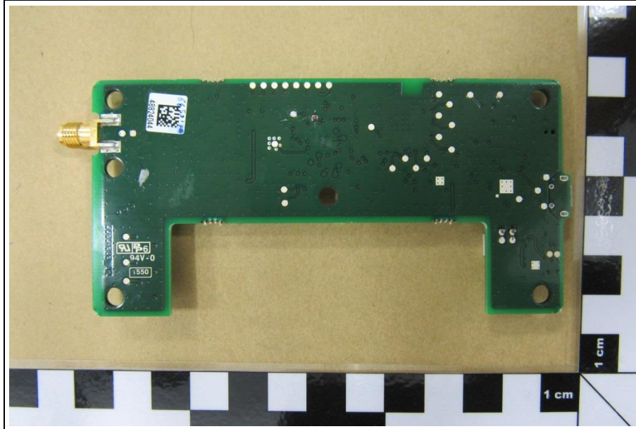
PCB BOTTOM
