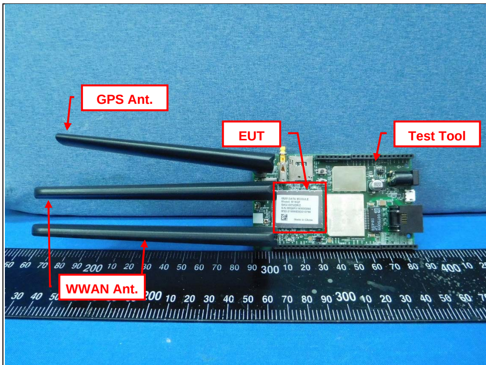
Antenna + EUT + Test Tool
