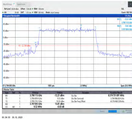
1-N78-3700-3800-30-10-H-3-DFT-16QAM-Outer_Ful I-24@0-Ant1-8.575-9.520-≤10-PASS
