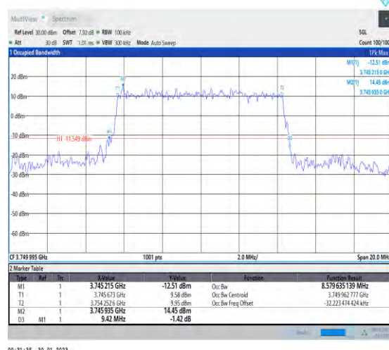
1-N78-3700-3800-30-10-M-3-DFT-16QAM-Outer_Ful I-24@0-Ant1-8.58-9.420-≤10-PASS
