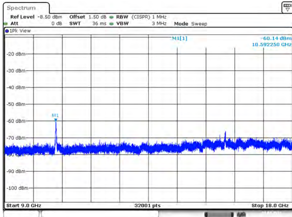
Plot on IEEE 802.11ac Nss1 MCS0 VHT20 / 5300 MHz / Peak / Port 1 / 9GHz~18GHz
