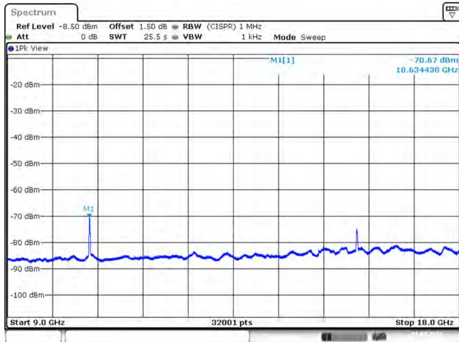
Plot on IEEE 802.11ac Nss1 MCS0 VHT20 / 5320 MHz / Average / Port 2 / 9GHz~18GHz
