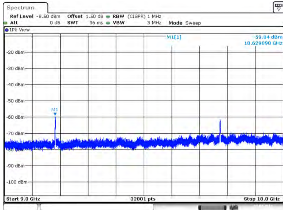
Plot on IEEE 802.11ac Nss1 MCS0 VHT20 / 5320 MHz / Peak / Port 2 / 9GHz~18GHz
