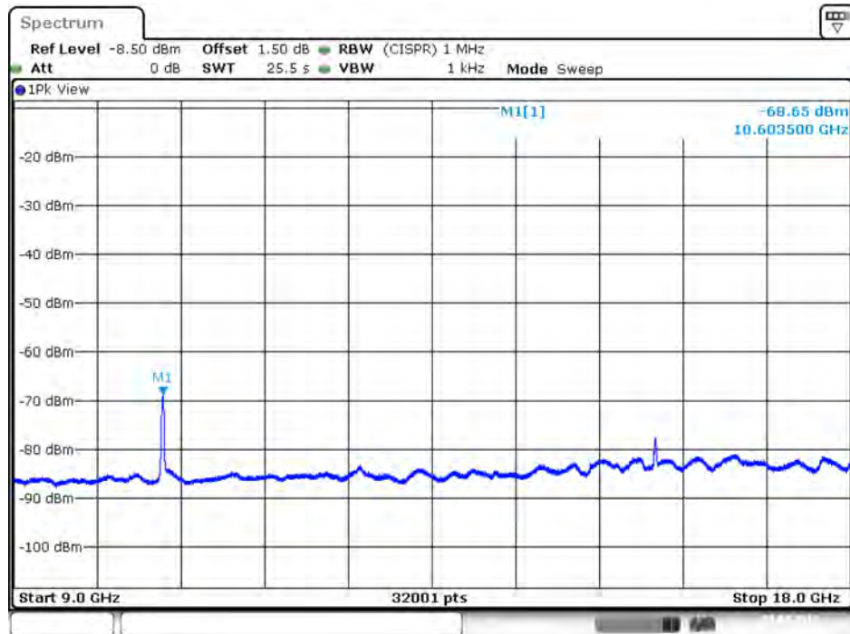
Plot on IEEE 802.11ac Nss1 MCS0 VHT20 / 5300 MHz / Average / Port 1 / 9GHz~18GHz
