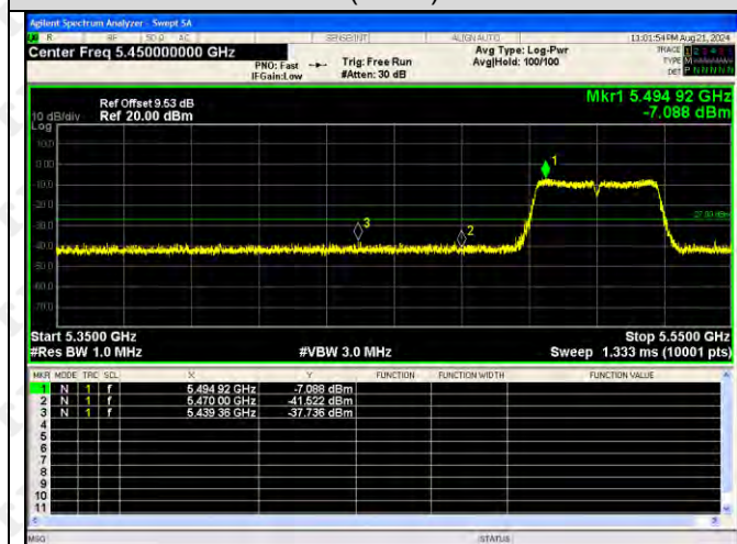
802.11ac(VH80)-5530
