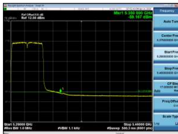
5310MHz with 4*4 Beamforming AV
