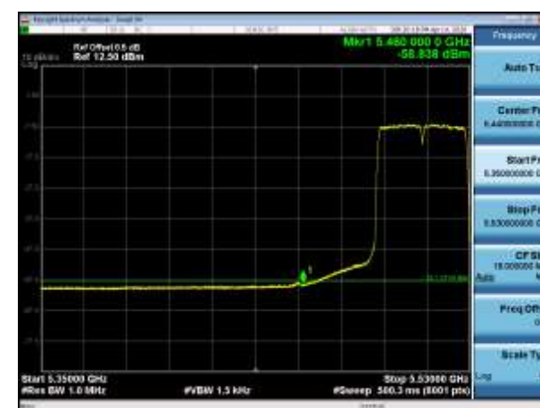
5510MHz with 4*4 Beamforming AV
