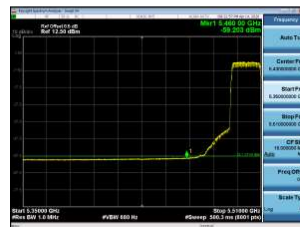
5500MHz with 4*4 Beamforming AV
