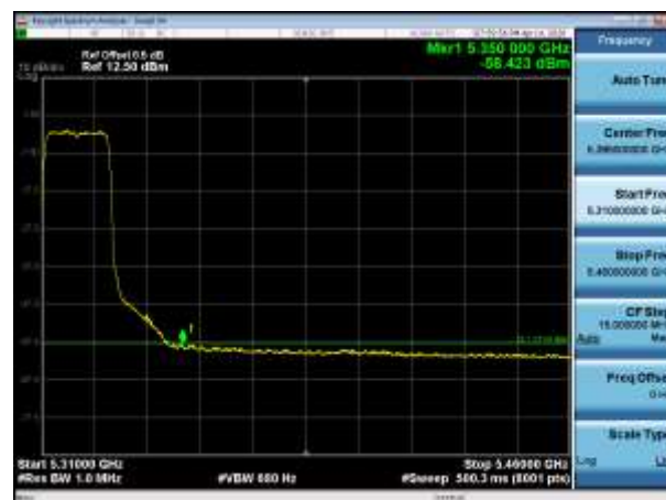
5320MHz with 4*4 Beamforming AV
