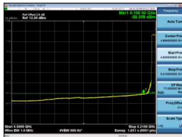
5200MHz with 4*4 Beamforming AV
