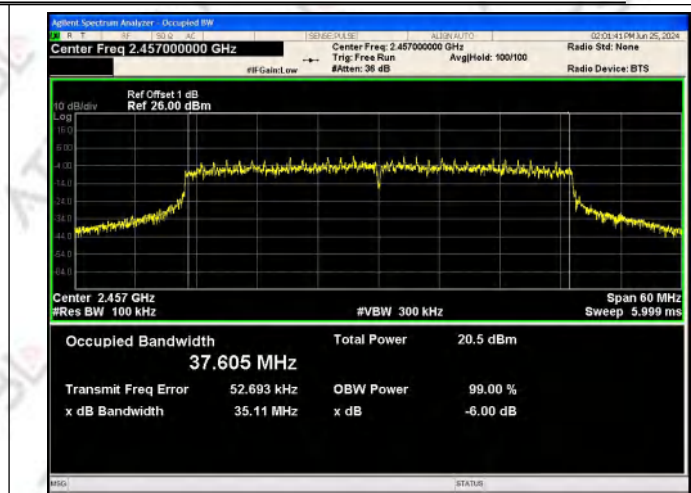
IEEE 802.11ax_Channel 10_40MHz_Antenna 0_RU&Index SU
