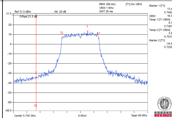
802.11a / Chain 3 : CH149
