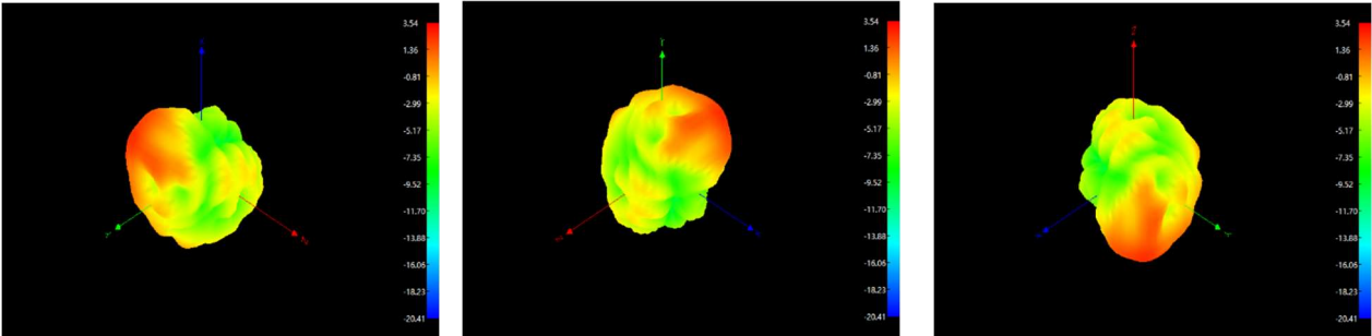
Antenna 3D 5500MHz:
