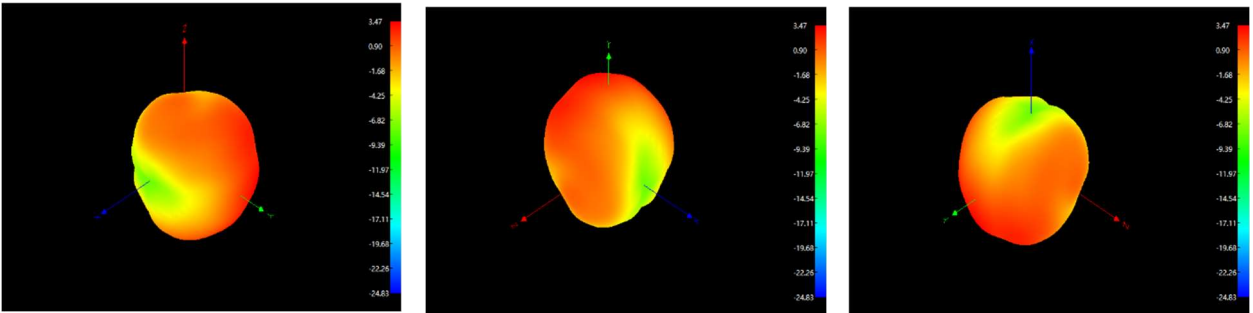
Antenna 3D 2500MHz:
