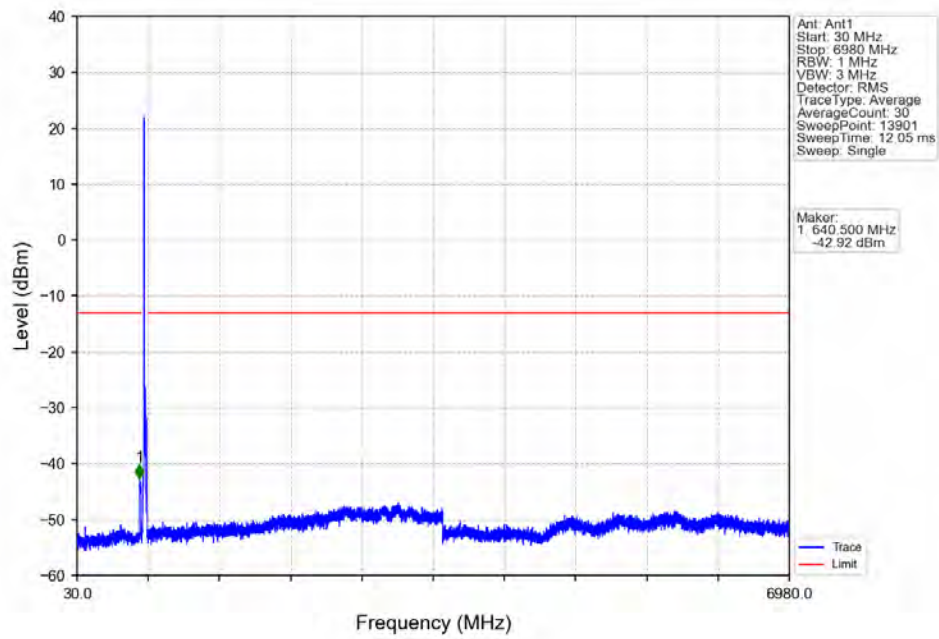
Band71_15MHz_QPSK_HCH_690.5MHz_RB_1_74_NTNV
