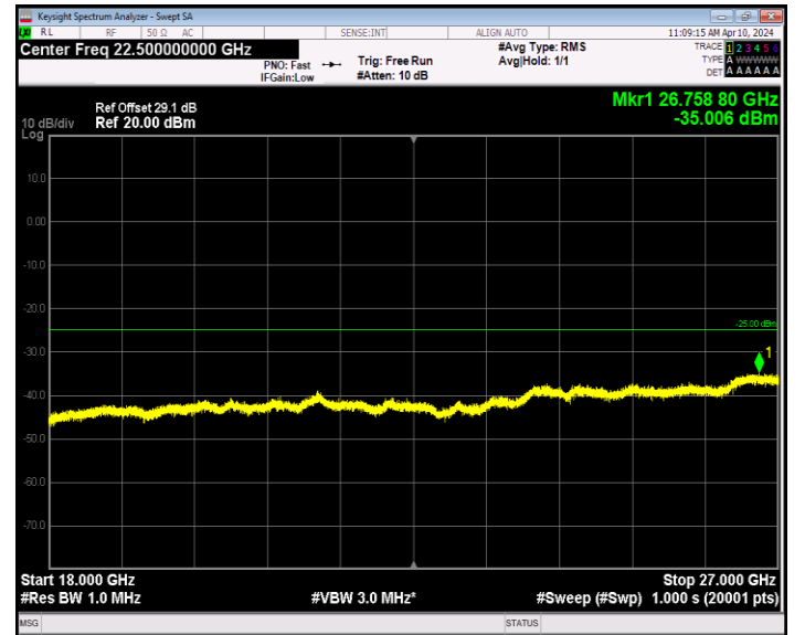
Band7_20MHz_QPSK_21350_1RB#0_18000~27000_18000~27000
