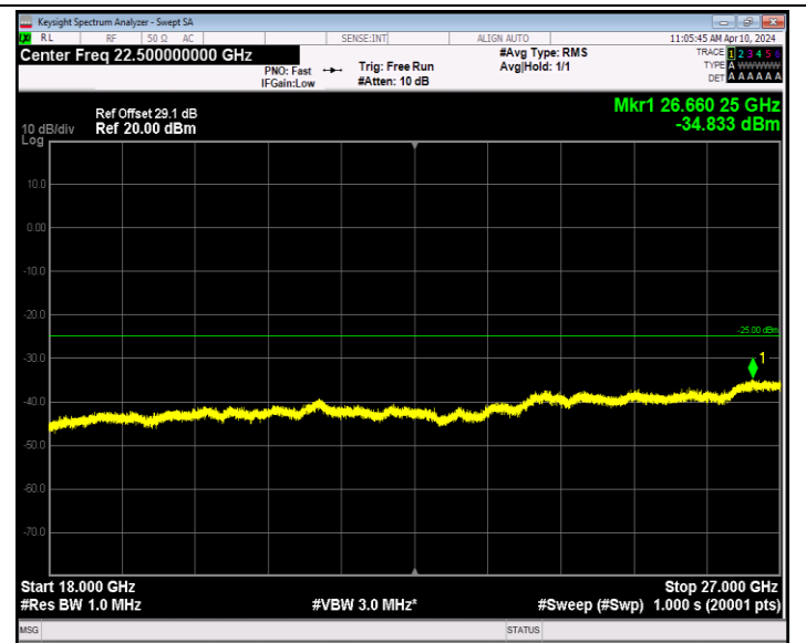
Band7_20MHz_QPSK_20850_1RB#0_18000~27000_18000~27000
