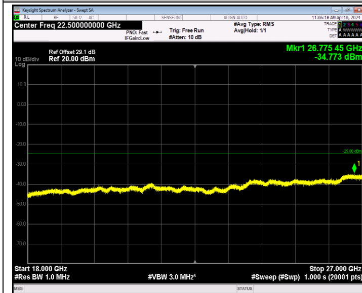
Band7_20MHz_16QAM_20850_1RB#0_18000~27000_18000~27 000
