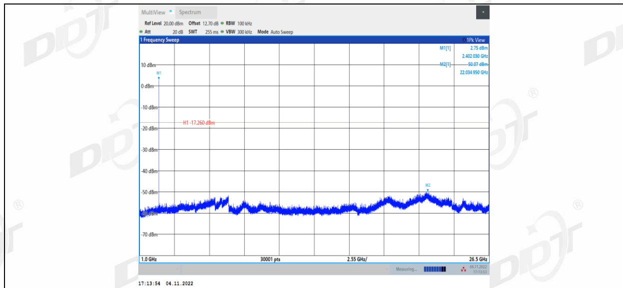
BLE 2M_Ant1_2440_0~Reference
