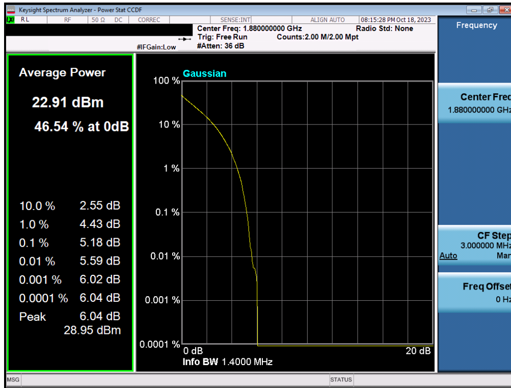
Plot 7-56. PAR Plot (LTE Band 2 - 1.4MHz QPSK - Full RB - Ant2)
