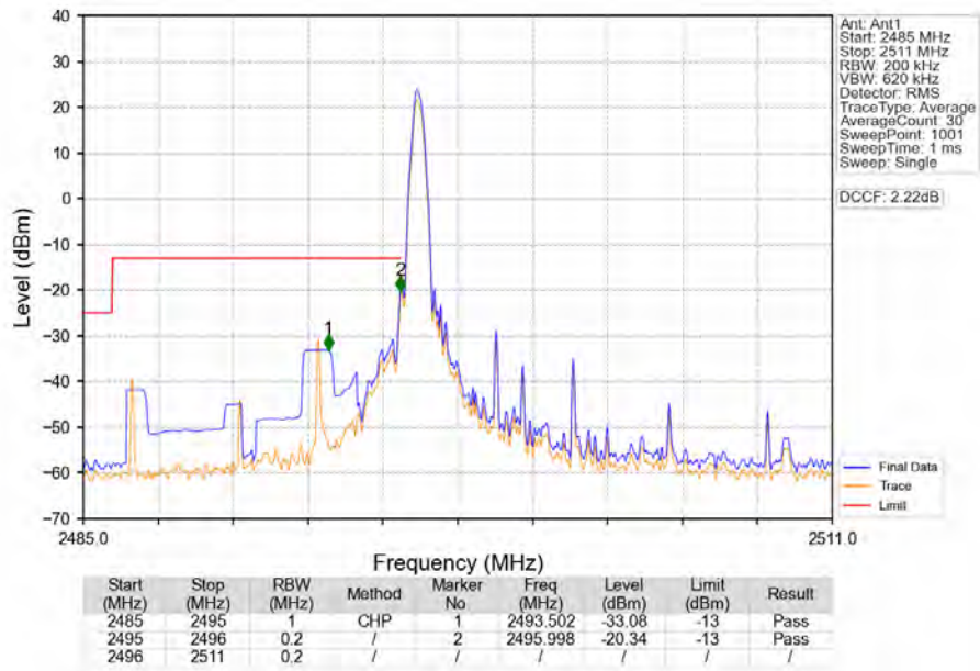
Band41_10MHz_QPSK_LCH_2501MHz_RB_1_0_NTNV
