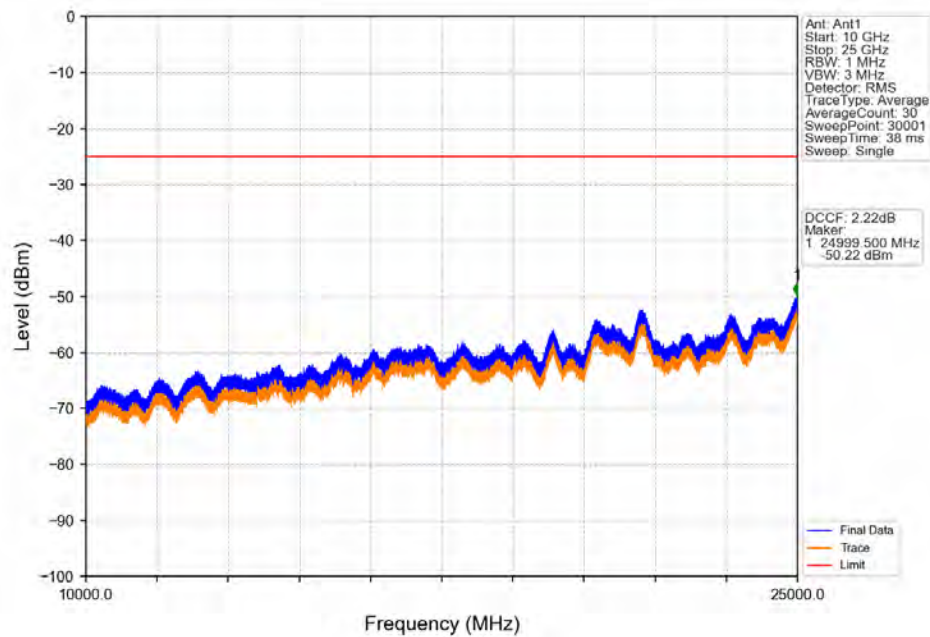
Band41_5MHz_QPSK_LCH_2498.5MHz_RB_1_0_NTV
