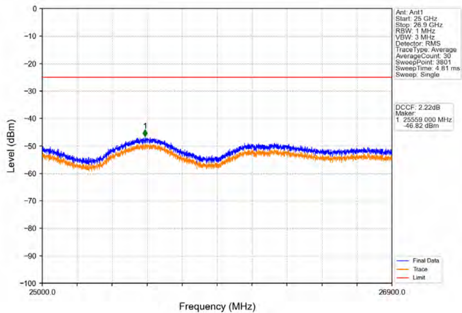
Band41_5MHz_QPSK_LCH_2498.5MHz_RB_1_0_NTV
