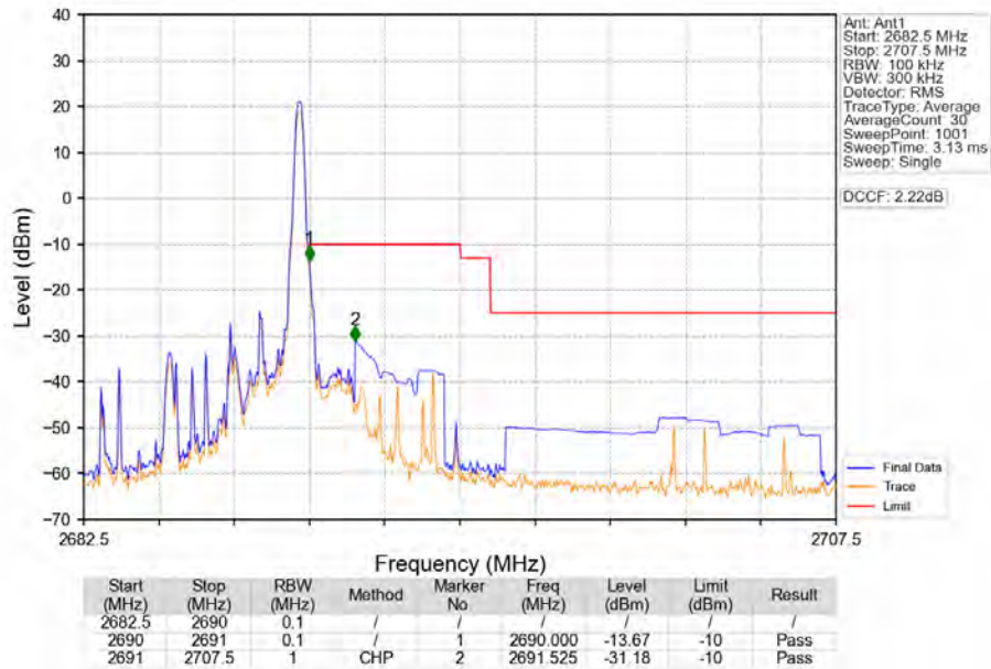
Band41_5MHz_QPSK_HCH_2687.5MHz_RB_1_24_NTV
