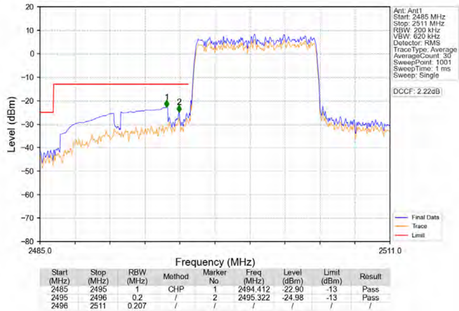
Band41_10MHz_16QAM_LCH_2501MHz_RB_50_0_NTNV
