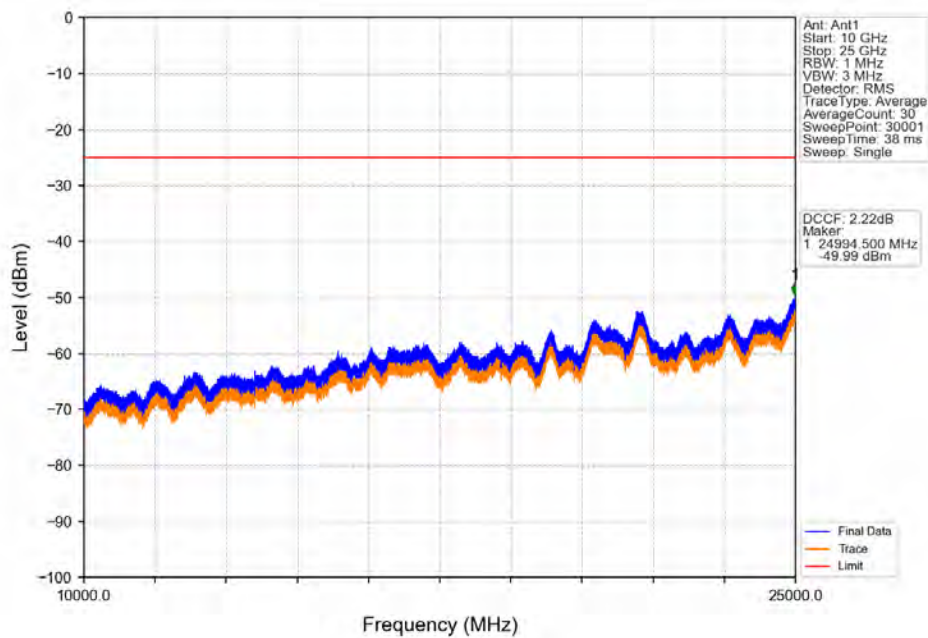
Band41_10MHz_16QAM_MCH_2593MHz_RB_1_0_NTNV
