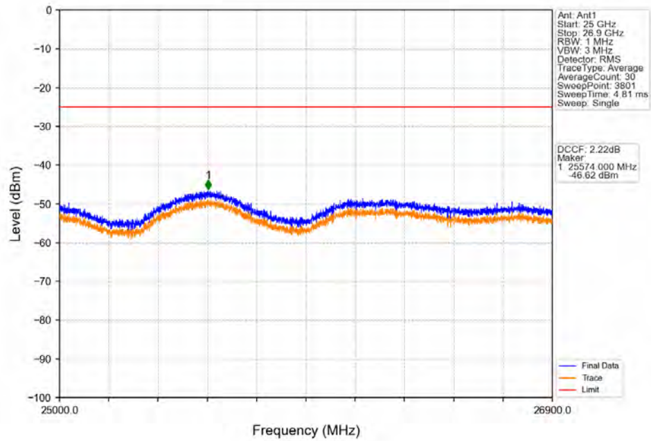
Band41_5MHz_QPSK_HCH_2687.5MHz_RB_1_24_NTV
