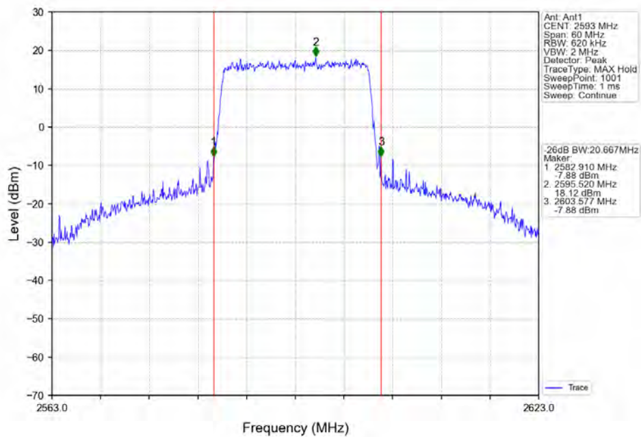
Band41_20MHz_16QAM_MCH_2593MHz_RB_100_0 NTN
