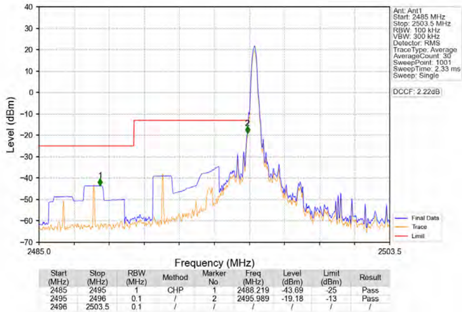
Band41_5MHz_16QAM_LCH_2498.5MHz_RB_1_0 NTN
