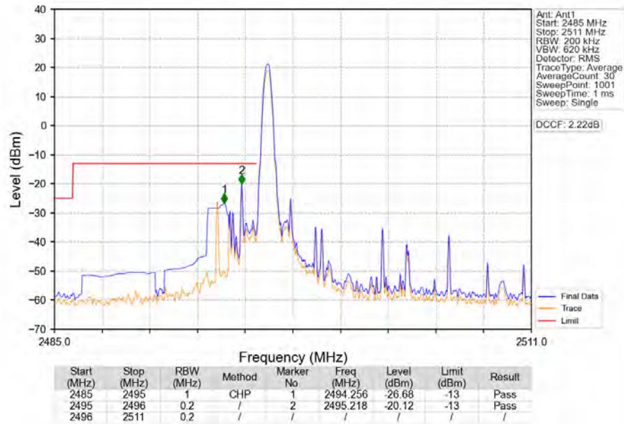
Band41_10MHz_16QAM_LCH_2501MHz_RB_1_0_NTNV
