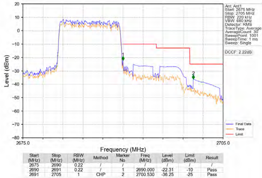
Band41_10MHz_QPSK_HCH_2685MHz_RB_50_0_NTNV
