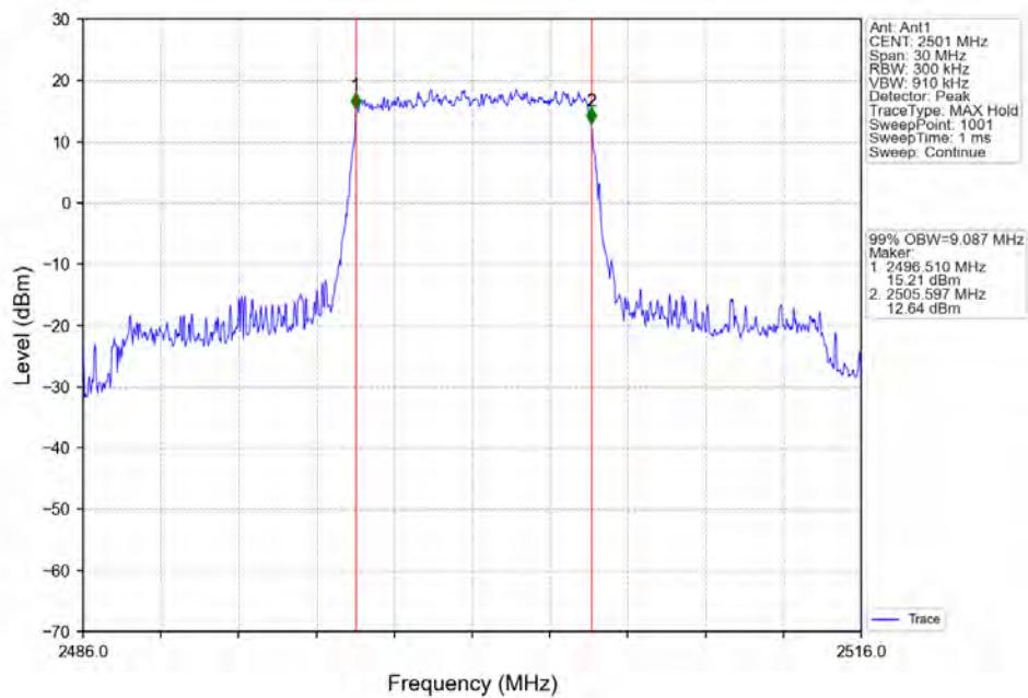
Band41_10MHz_QPSK_LCH_2501MHz_RB_50_0 NTN
