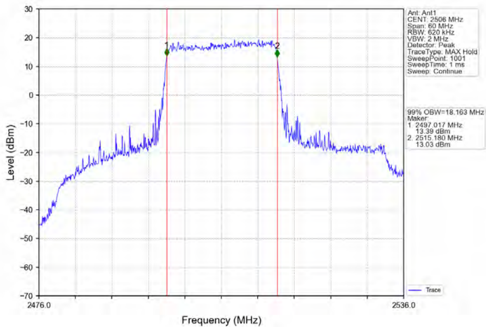
Band41_20MHz_QPSK_LCH_2506MHz_RB_100_0_NTN
