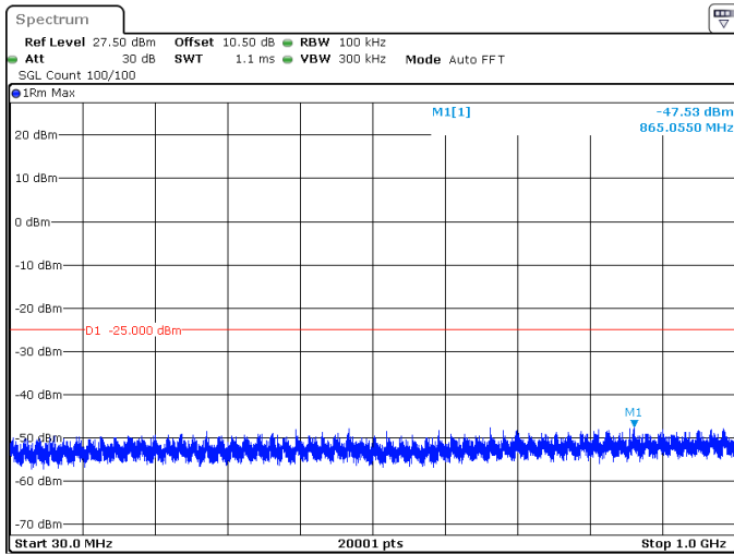
20MHz_15kHz_2679.99MHz_DFT-s-OFDM QPSK_RB1@105 -47.53 dBm
