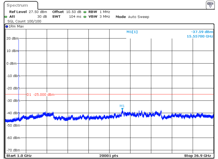
20MHz_15kHz_2679.99MHz_DFT-s-OFDM QPSK_RB1@0 -37.59 dBm
