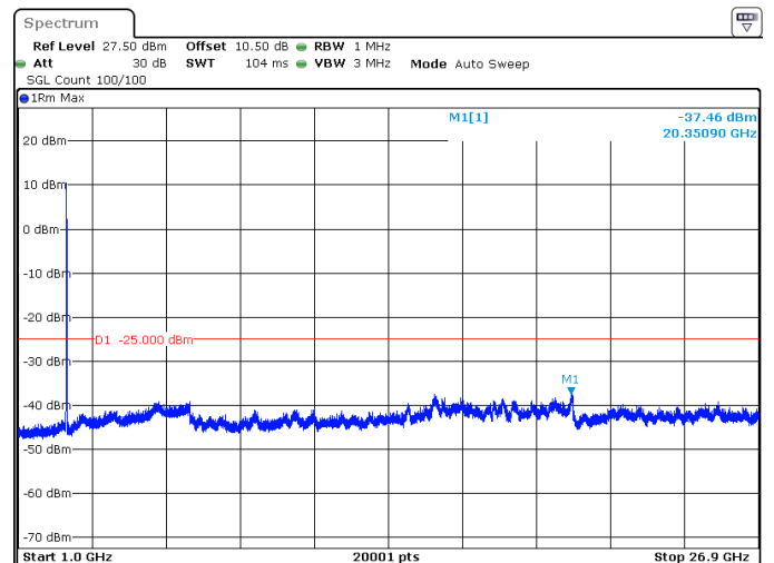
20MHz_15kHz_2679.99MHz_DFT-s-OFDM QPSK_RB100@0 -37.46 dBm
