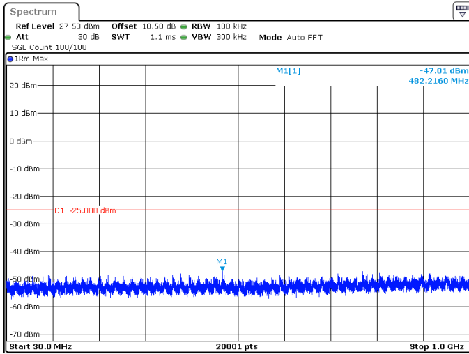
20MHz_15kHz_2679.99MHz_DFT-s-OFDM QPSK_RB1@0 -47.01 dBm
