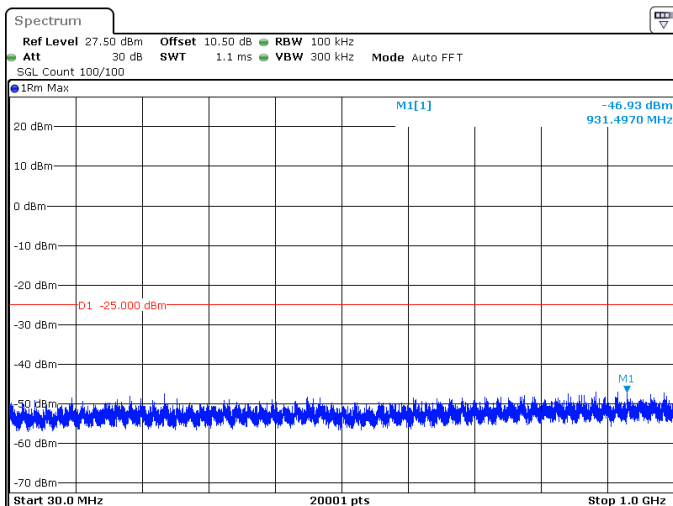
20MHz_15kHz_2679.99MHz_DFT-s-OFDM QPSK_RB100@0 -46.93 dBm
