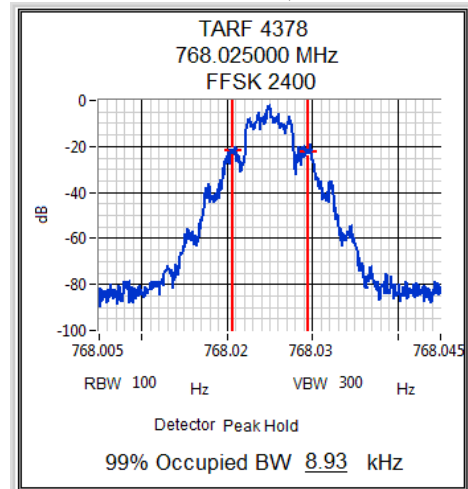
768.025 MHz, 3 W
