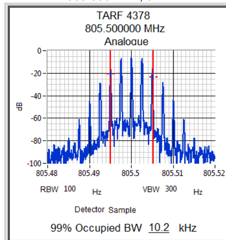
805.500 MHz, 3 W
