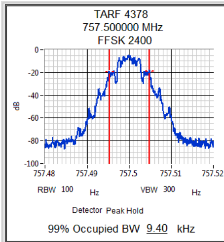
757.500 MHz, 3 W
