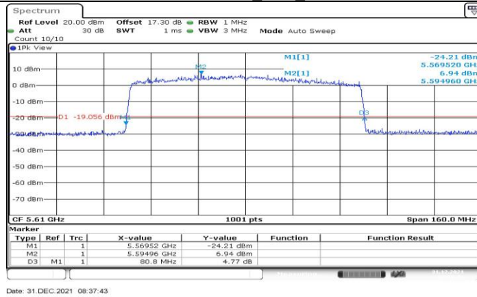
11AX80MIMO Ant1 5610
