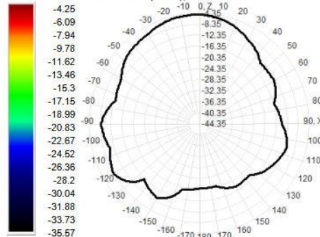
2450.0MHz Total(E1-XZ), Max=-4.84dBi
