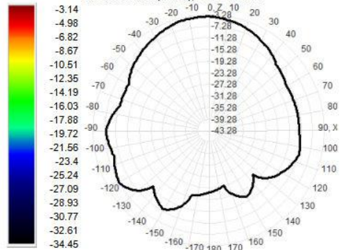
2400.0MHz Total(E1-XZ), Max=-3.94dBi
