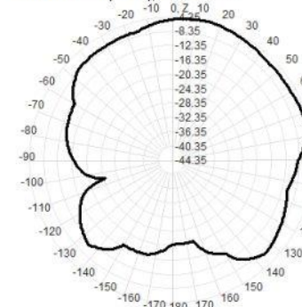
2450.0MHz Total(E2-YZ), Max=-4.35dBi
