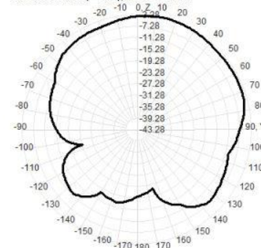
2400.0MHz Total(E2-YZ), Max=-3.28dBi
