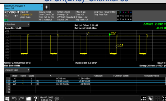
\pi/4 DQPSK(2-DH5)_Channel 0
