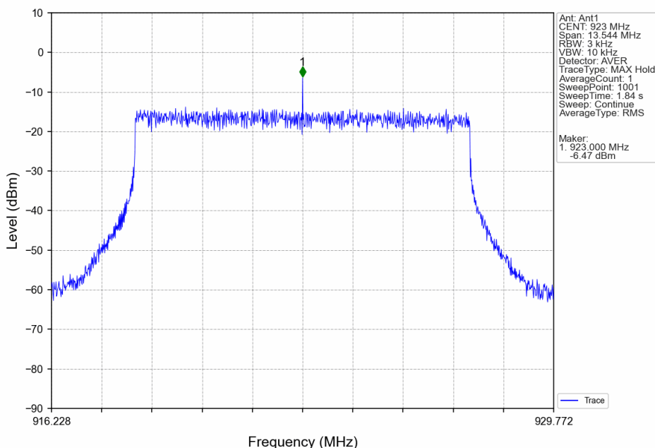
10M_HCH_923MHz_MIMO_NTNV
