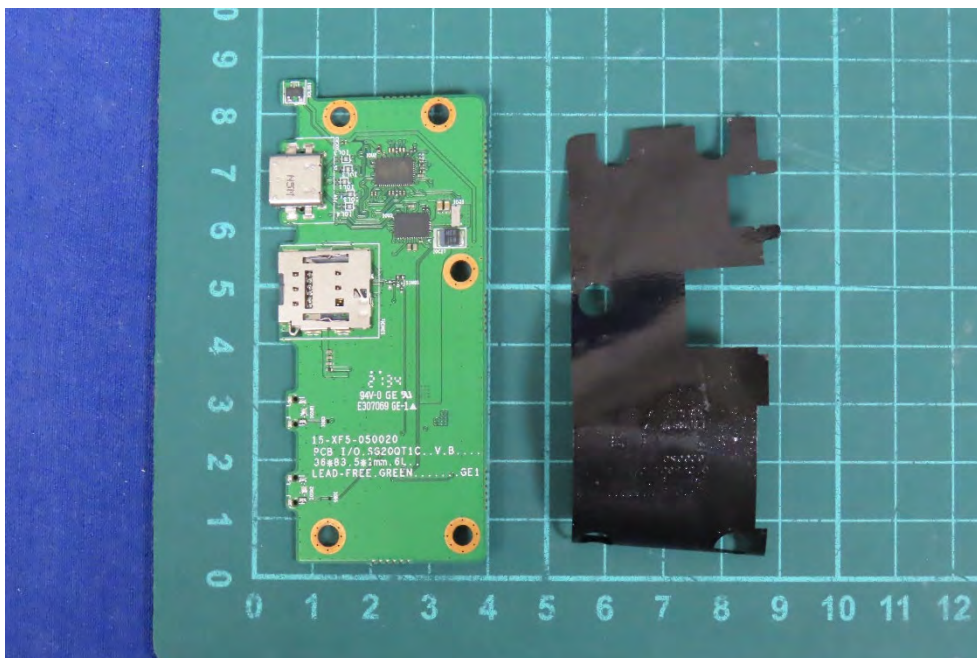
(13) EUT Photo
