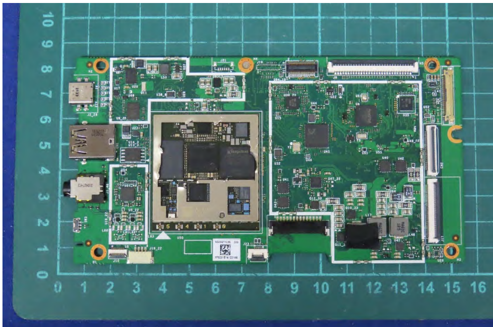
(21) EUT Photo
