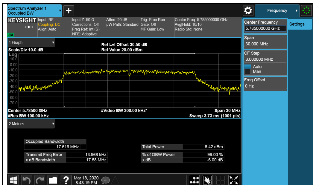
802.11n-HT20-5785MHz
