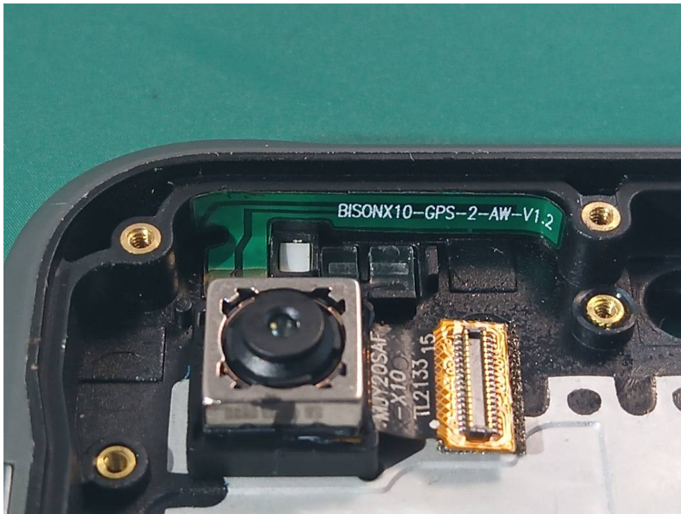
GPS Antenna
