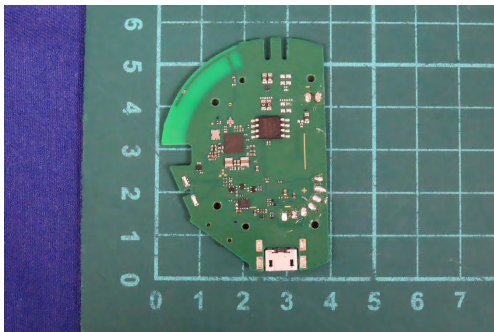
(49) EUT Photo
