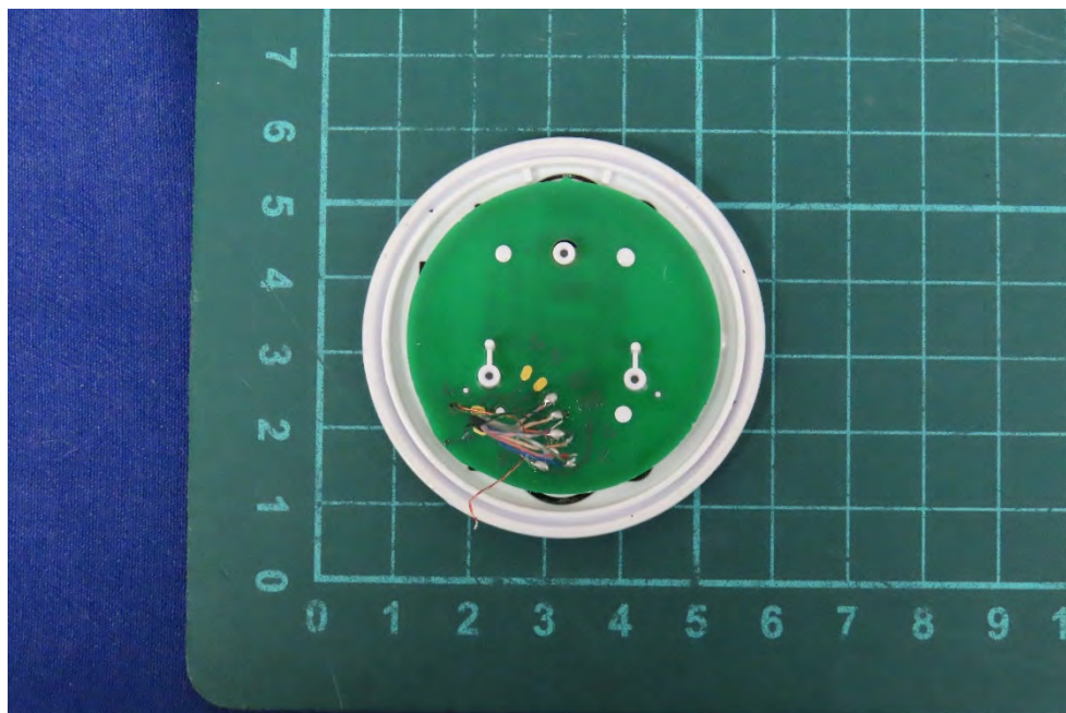
(54) EUT Photo
