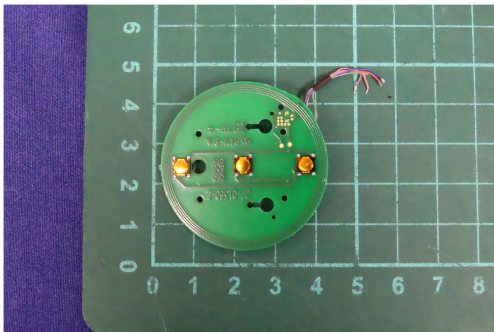
(57) EUT Photo
