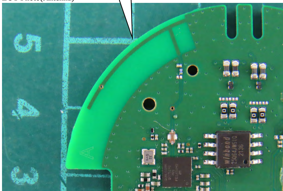
(30) EUT Photo(Antenna)
