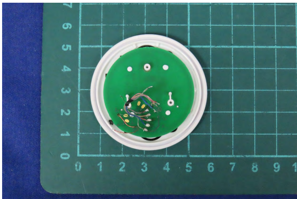
(33) EUT Photo
