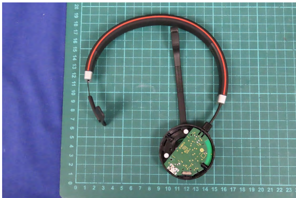
(46) EUT Photo
