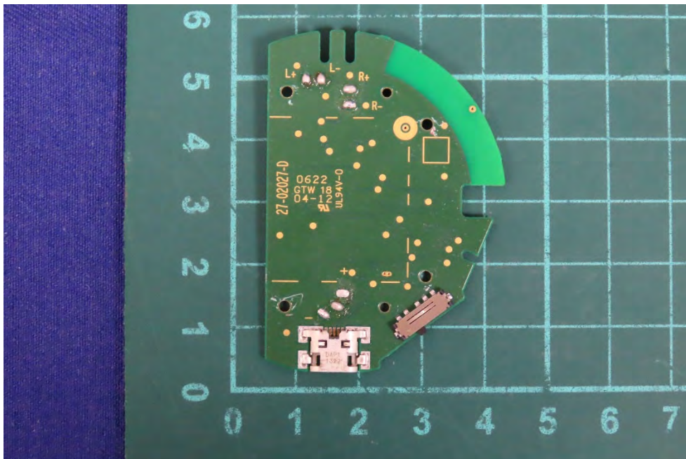
(48) EUT Photo
