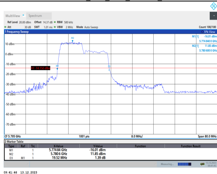
11AX40MIMO_Ant2_5795_242Tone_RU61
