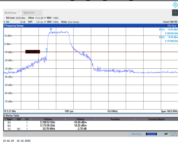
11AX80MIMO_Ant1_5210_484Tone_RU65
