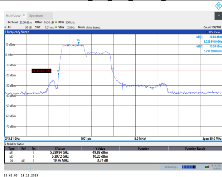
11AX40MIMO_Ant2_5310_242Tone_RU61
