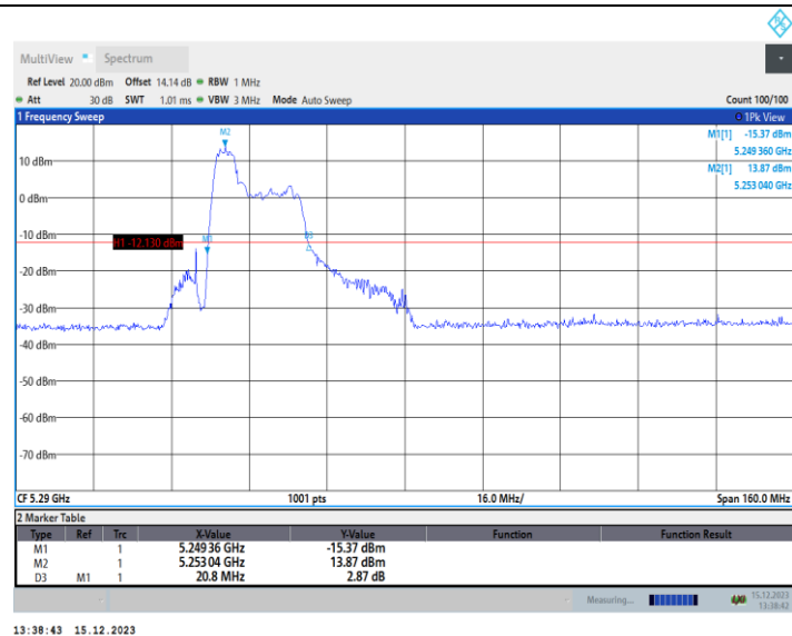
11AX80MIMO_Ant1_5290_106Tone_RU53
