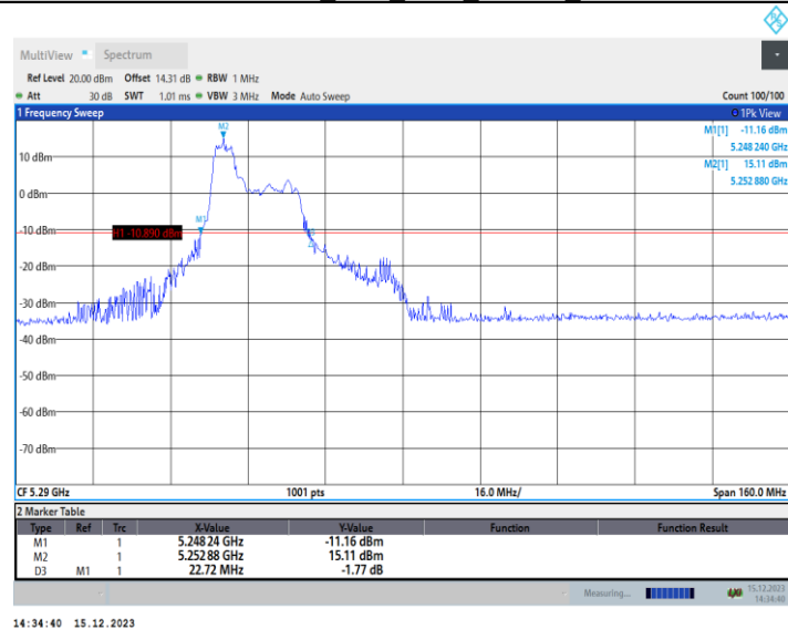
11AX80MIMO_Ant2_5290_106Tone_RU53
