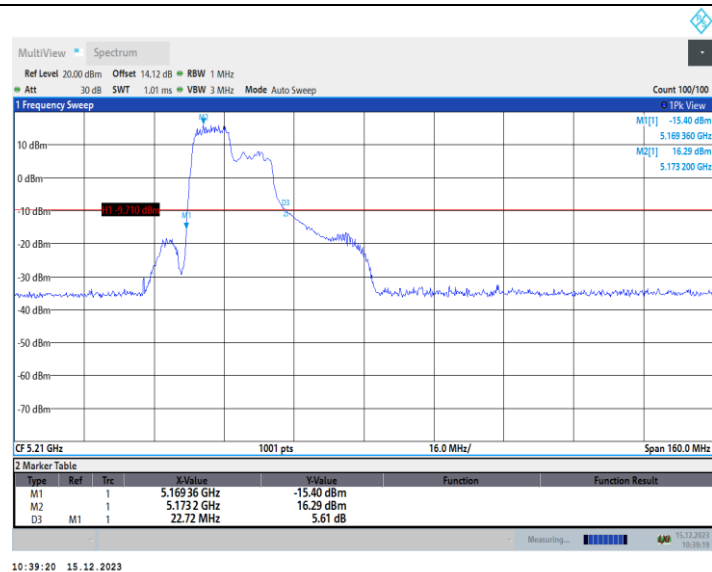
11AX80MIMO_Ant1_5210_242Tone_RU64
