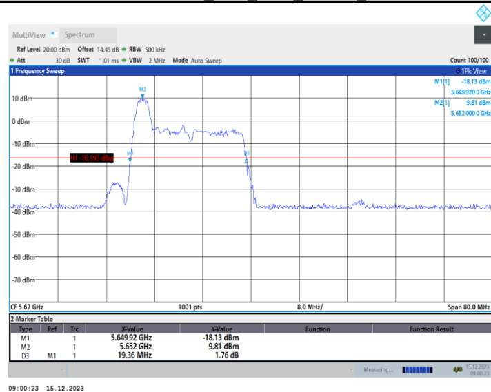
11AX40MIMO_Ant1_5670_52Tone_RU37
