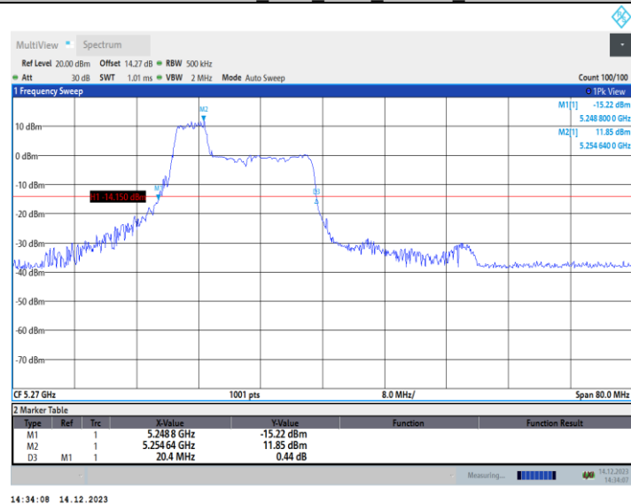
11AX40MIMO_Ant2_5270_106Tone_RU53
