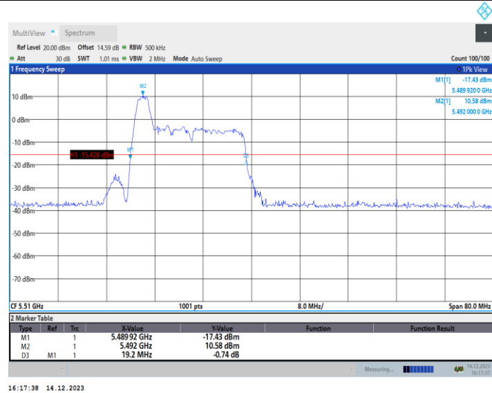
11AX40MIMO_Ant2_5510_52Tone_RU37
