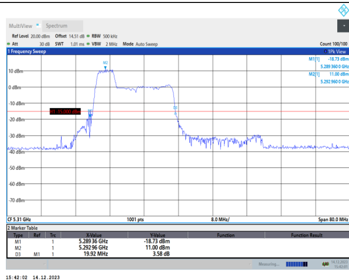
11AX40MIMO_Ant2_5310_106Tone_RU53
