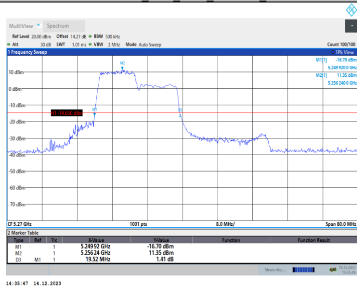
11AX40MIMO_Ant2_5270_242Tone_RU61
