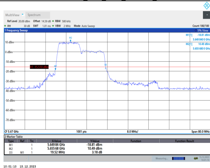
11AX40MIMO_Ant2_5670_242Tone_RU61
