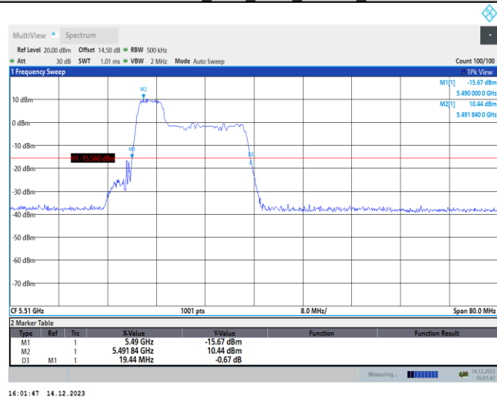
11AX40MIMO_Ant1_5510_106Tone_RU53
