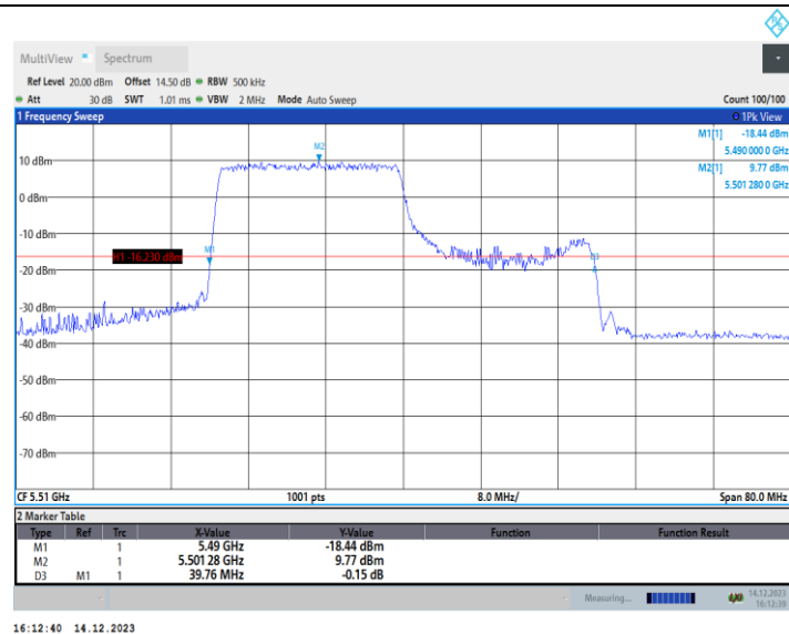
11AX40MIMO_Ant2_5510_26Tone_RU0
