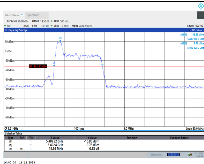
11AX40MIMO_Ant1_5510_52Tone_RU37
