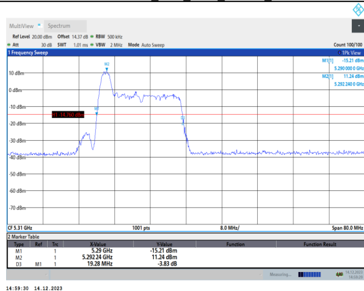
11AX40MIMO_Ant1_5310_52Tone_RU37
