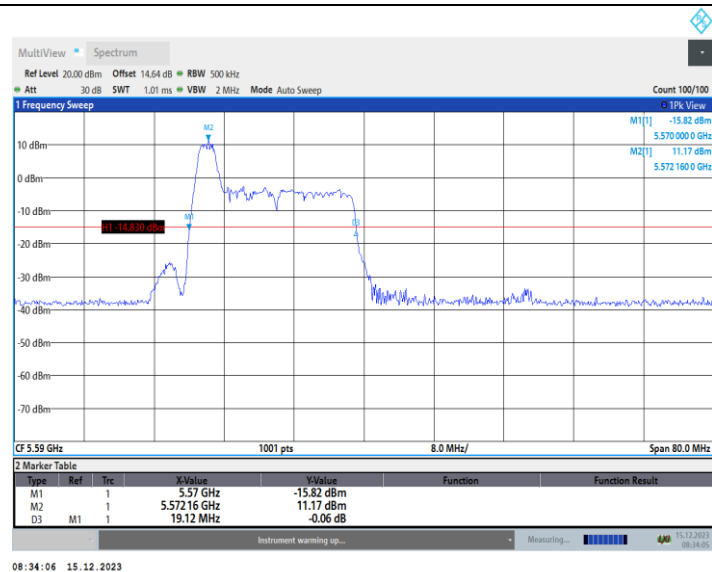
11AX40MIMO_Ant2_5590_52Tone_RU37
