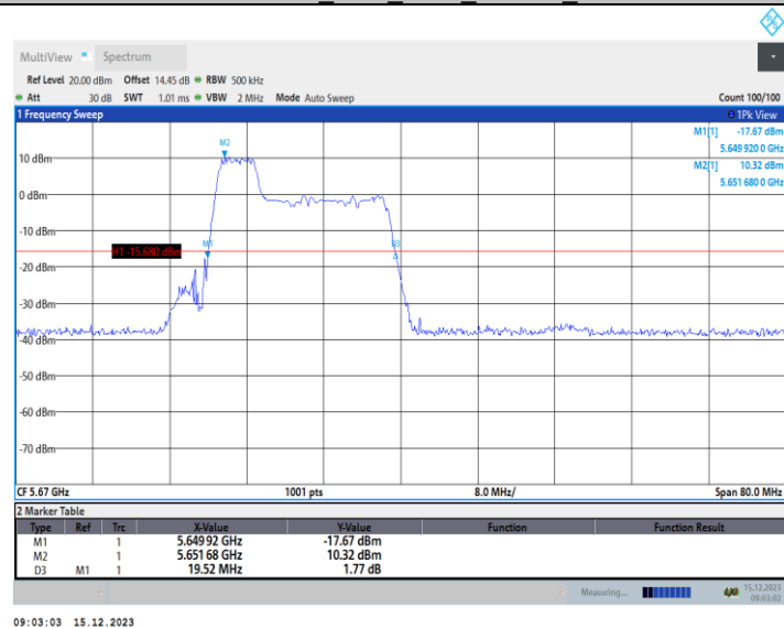
11AX40MIMO_Ant1_5670_106Tone_RU53
