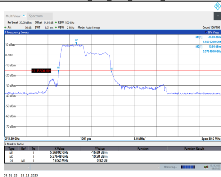
11AX40MIMO_Ant2_5590_242Tone_RU61
