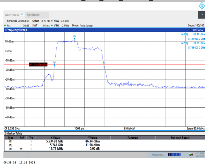
11AX40MIMO_Ant1_5755_242Tone_RU61
