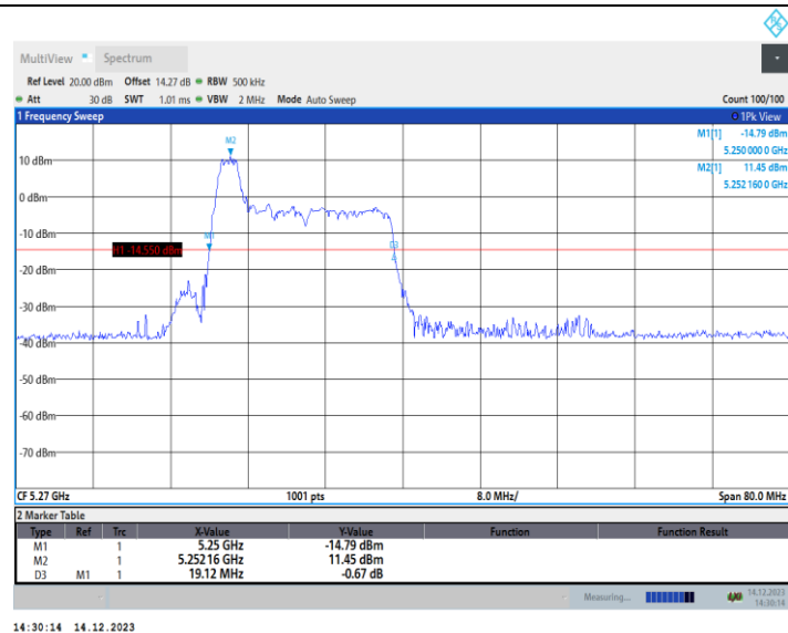
11AX40MIMO_Ant2_5270_52Tone_RU37
