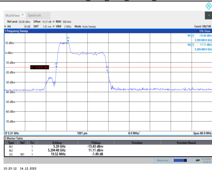
11AX40MIMO_Ant1_5310_106Tone_RU53
