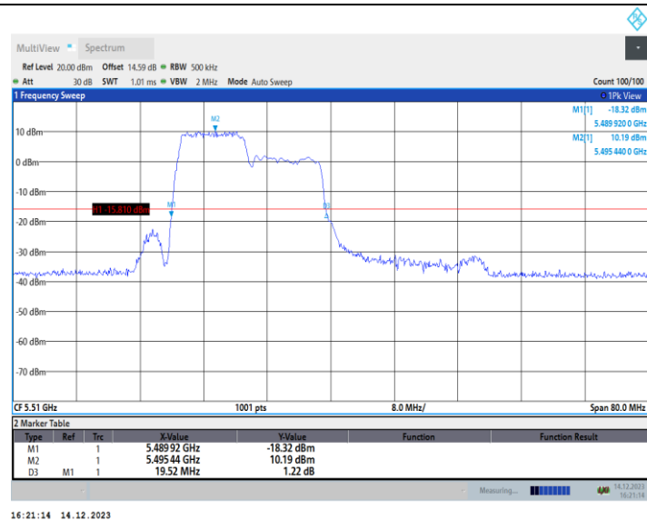
11AX40MIMO_Ant2_5510_242Tone_RU61
