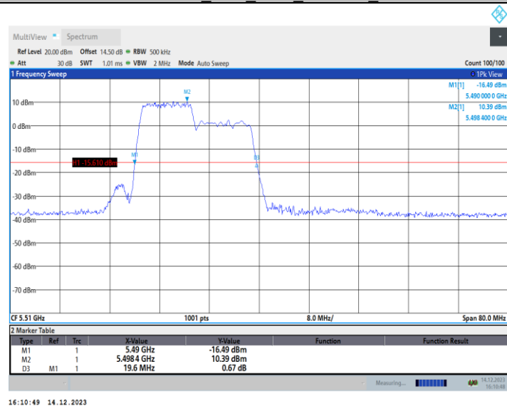
11AX40MIMO_Ant1_5510_242Tone_RU61
