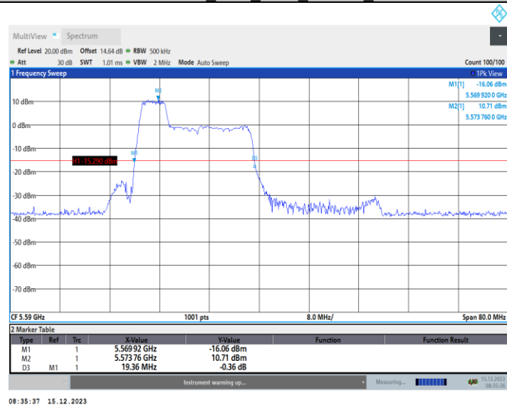
11AX40MIMO_Ant2_5590_106Tone_RU53
