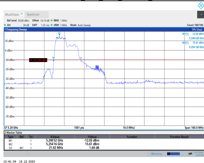
11AX80MIMO_Ant1_5290_242Tone_RU64
