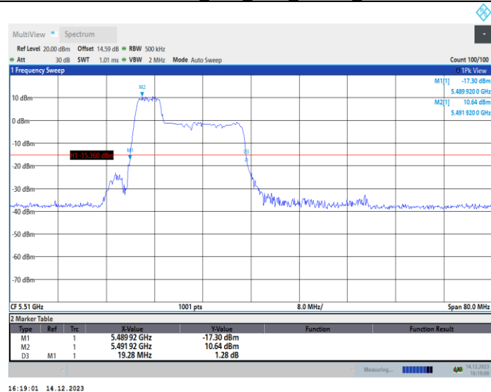
11AX40MIMO_Ant2_5510_106Tone_RU53
