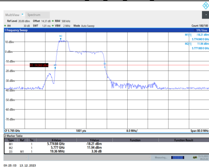
11AX40MIMO_Ant2_5795_106Tone_RU53
