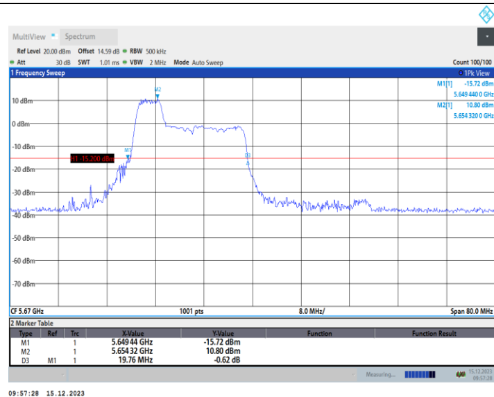
11AX40MIMO_Ant2_5670_106Tone_RU53
