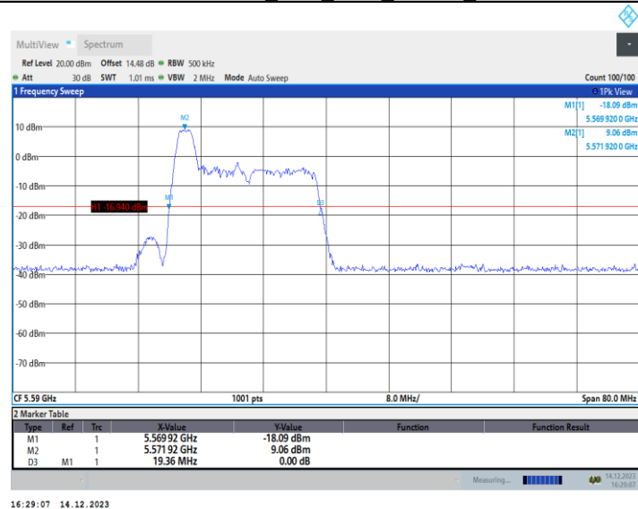
11AX40MIMO_Ant1_5590_52Tone_RU37
