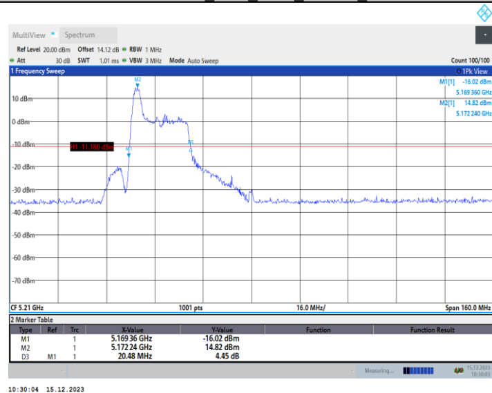
11AX80MIMO_Ant1_5210_52Tone_RU37
