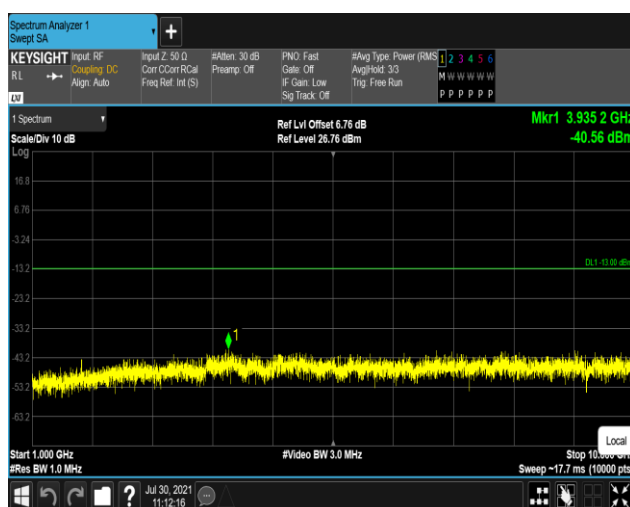
Band13-5MHz-QPSK-23230:1000~10000MHz
