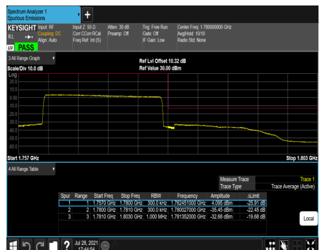
Band66-20MHz-QPSK-132572-100RB#0
