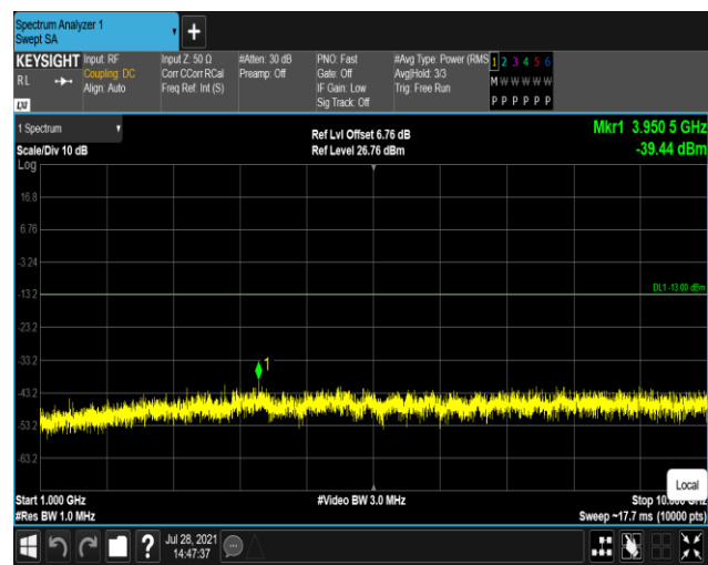
Band12-1.4MHz-QPSK-23095:1000~10000MHz
