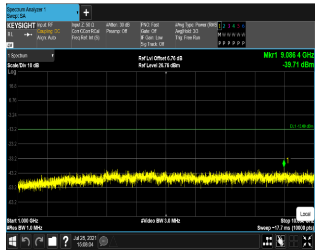
Band12-10MHz-QPSK-23095:1000~10000MHz
