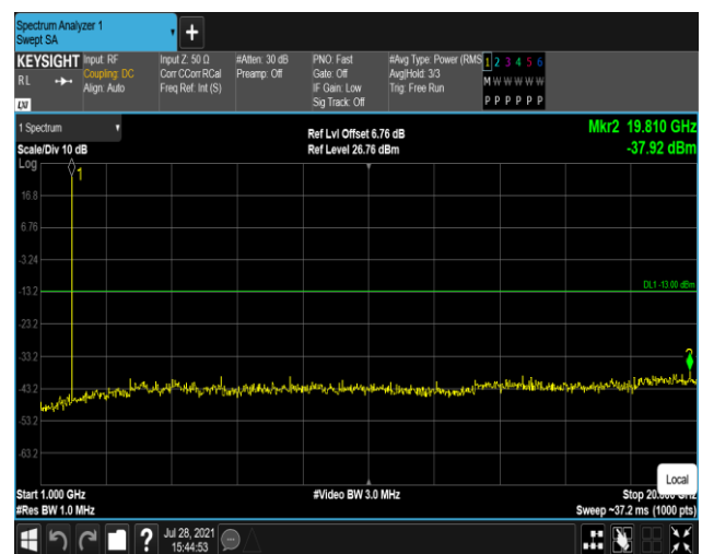
Band25-1.4MHz-QPSK-26683:1000~20000MHz
