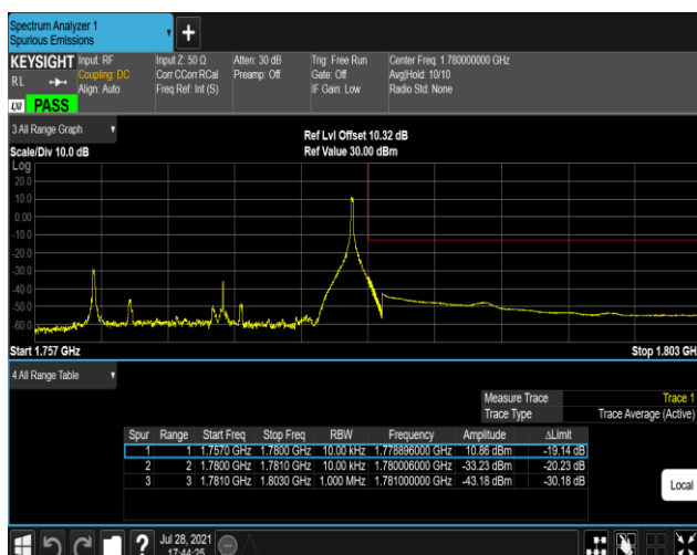
Band66-20MHz-QPSK-132572-1RB#99
