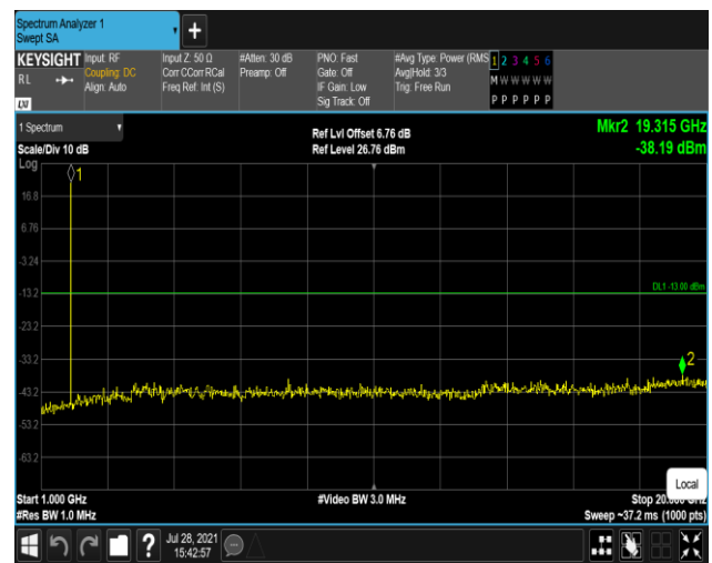
Band25-1.4MHz-QPSK-26365:1000~20000MHz
