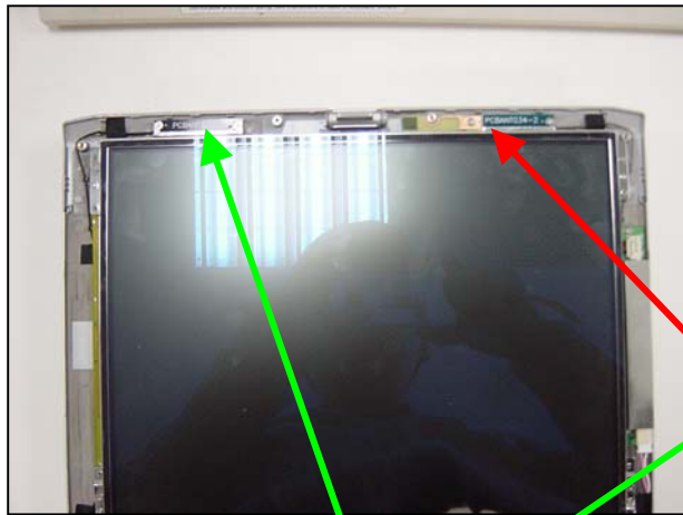
Aux(PIFA) Ant.
