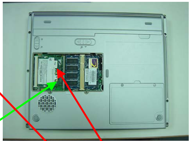
Main(PIFA) Ant.
