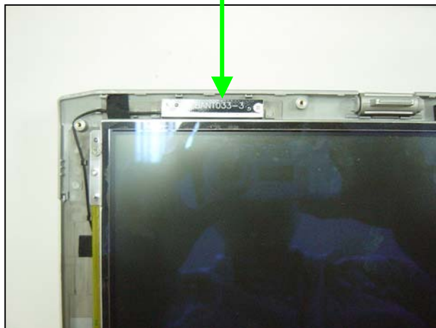
Aux(PIFA) Ant.
