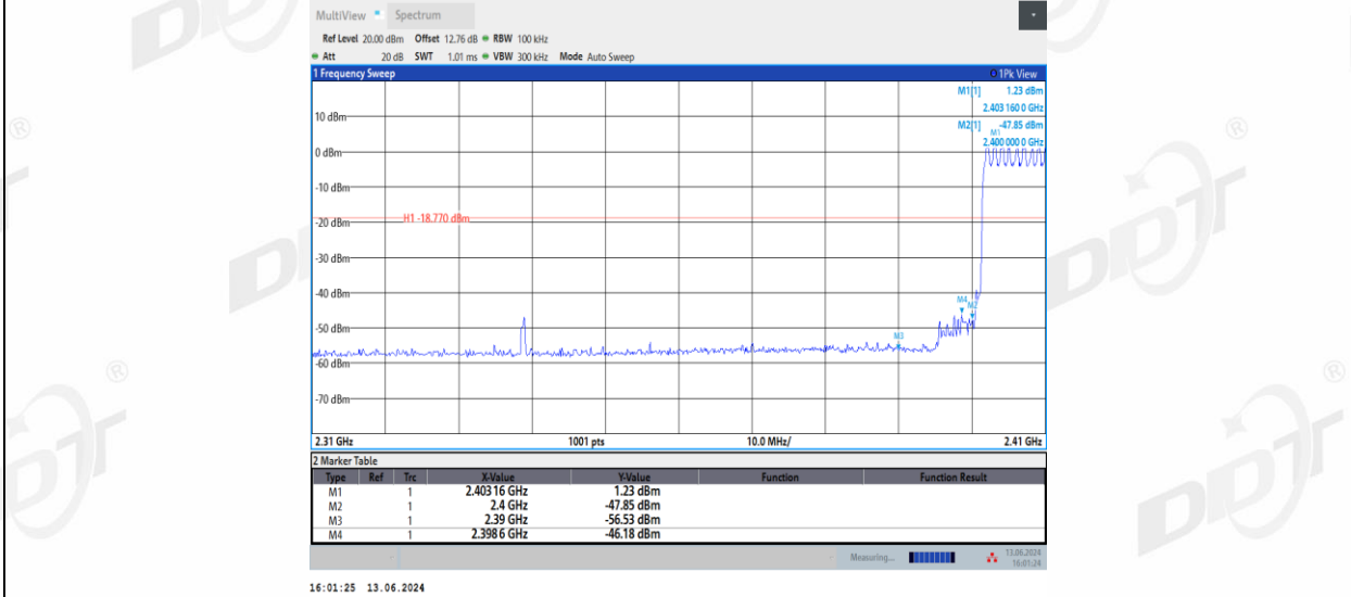
3DH5_Right side_Low_Hop_2402
