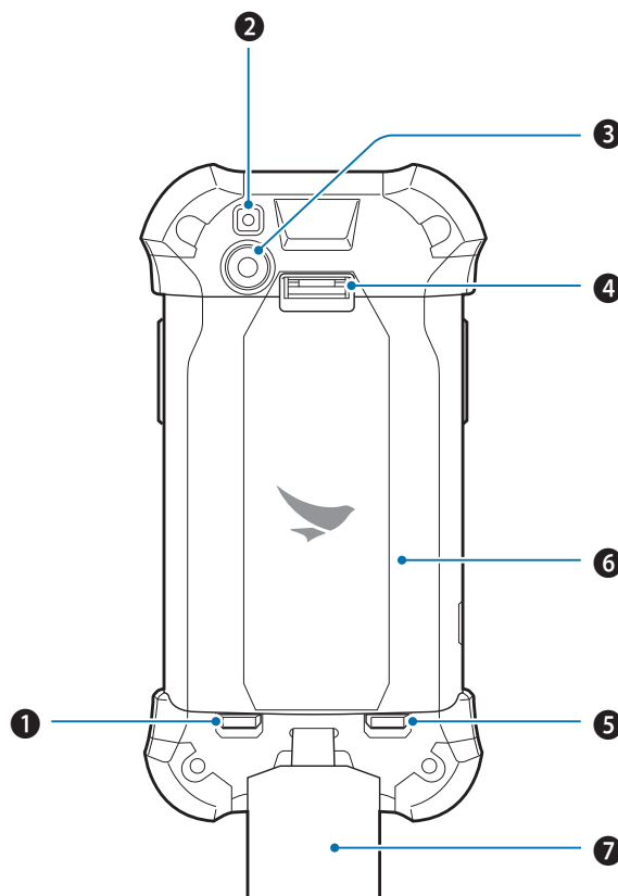
EF501R
