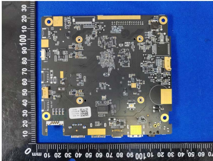
主板背面 (主板方案1) (适用于型号: SW2195T)
