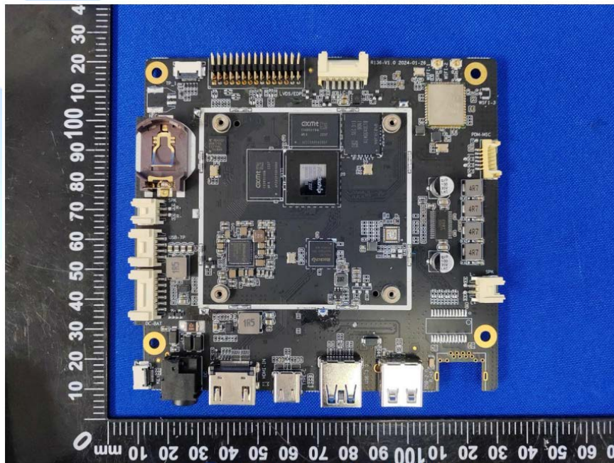
主板正面 (主板方案1) (适用于型号: SW2195T)
