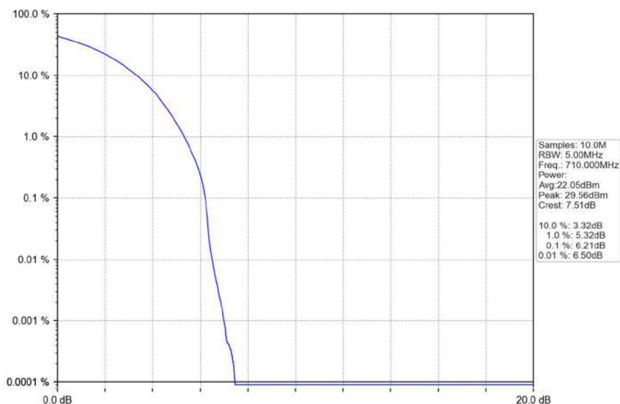
Band17_10MHz_QPSK_MCH_710MHz_RB_50_0_NTNV
