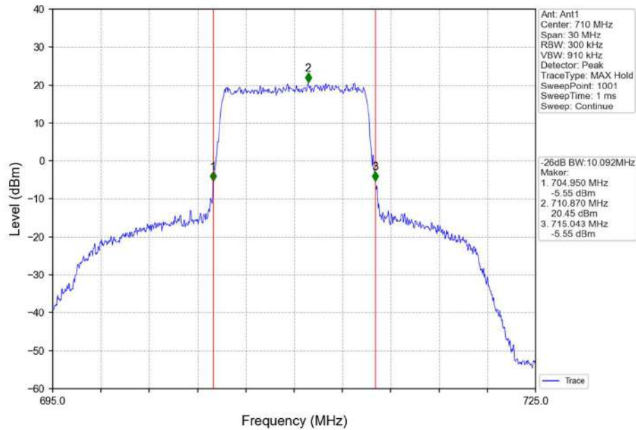
Band17_10MHz_QPSK_MCH_710MHz_RB_50_0_NTNV
