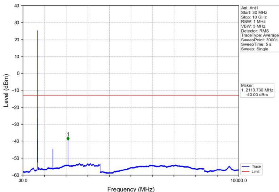
Band17_10MHz_QPSK_LCH_709MHz_RB_1_0_NTNV
