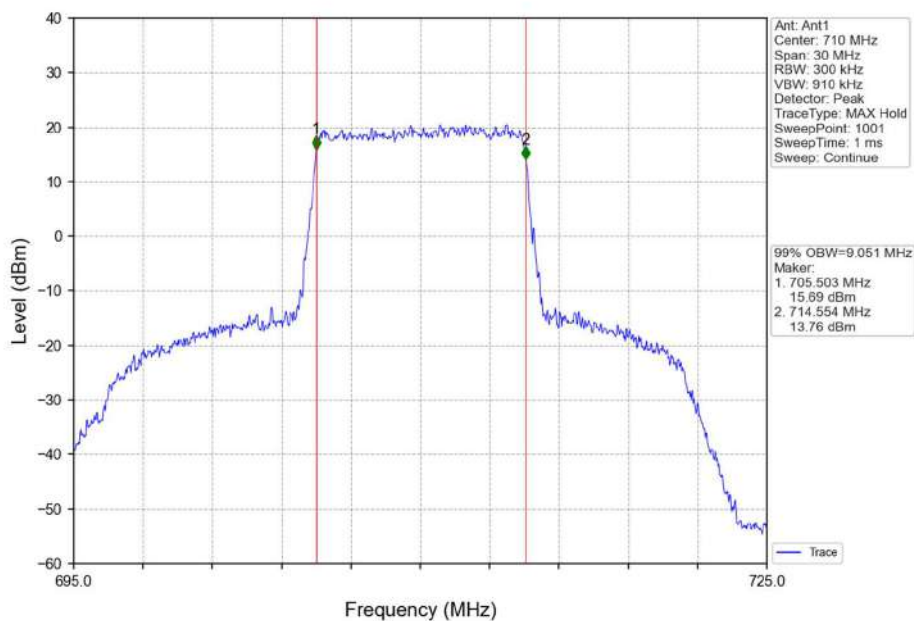
Band17_10MHz_QPSK_MCH_710MHz_RB_50_0_NTNV
