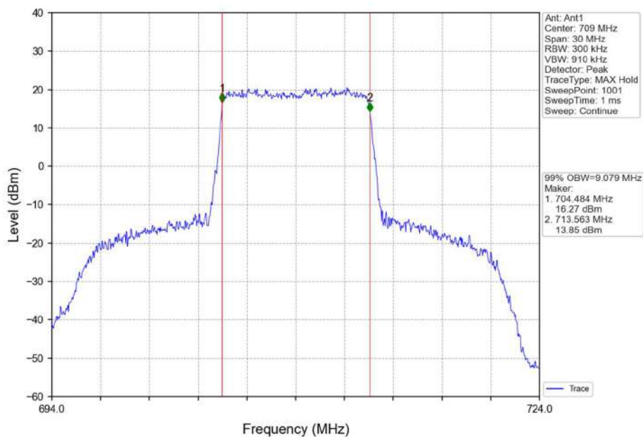
Band17_10MHz_QPSK_LCH_709MHz_RB_50_0_NTNV
