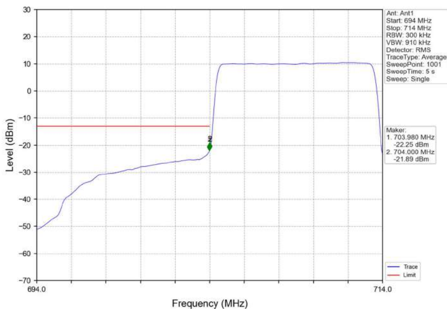
Band17 10MHz QPSK LCH 709MHz RB 50 0 NTV
