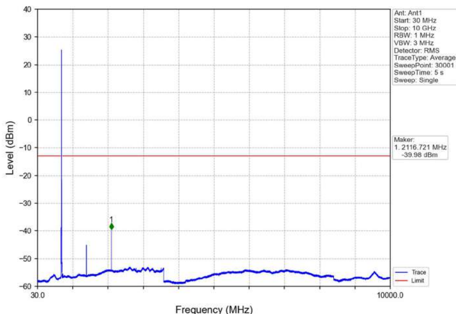
Band17_10MHz_QPSK_MCH_710MHz_RB_1_0_NTNV
