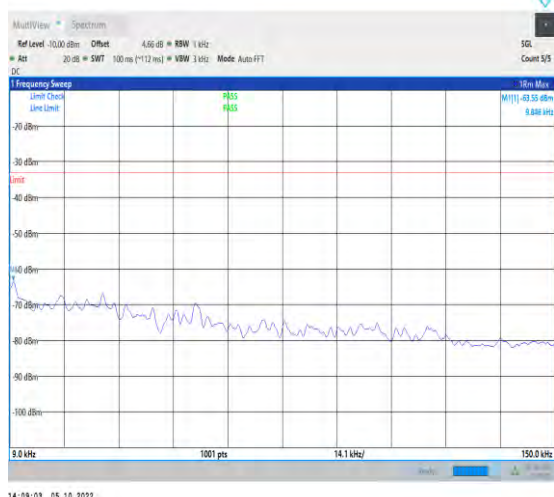
1-N71-PC3-15-20-L-1-DFT-QPSK-Inner_1RB_Left-1 @1-0.009-0.15-Ant1-0.01--63.55--33-PASS
