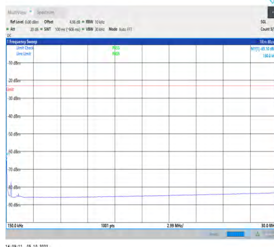
1-N71-PC3-15-20-L-1-DFT-QPSK-Inner_1RB_Left-1 @1-0.15-30-Ant1-0.15--65.10--23-PASS
