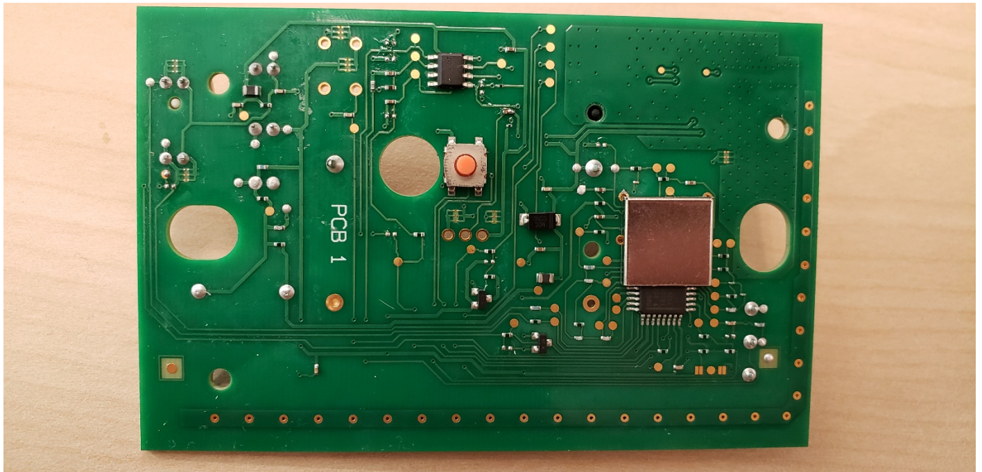
PCB BOTTOM
