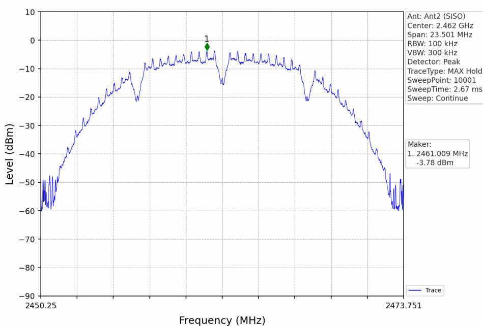
802.11g_HCH_2462MHz_Ant2 (SISO)_NTNV
