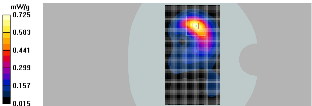
Fig.8 WCDMA1900 CH9538
