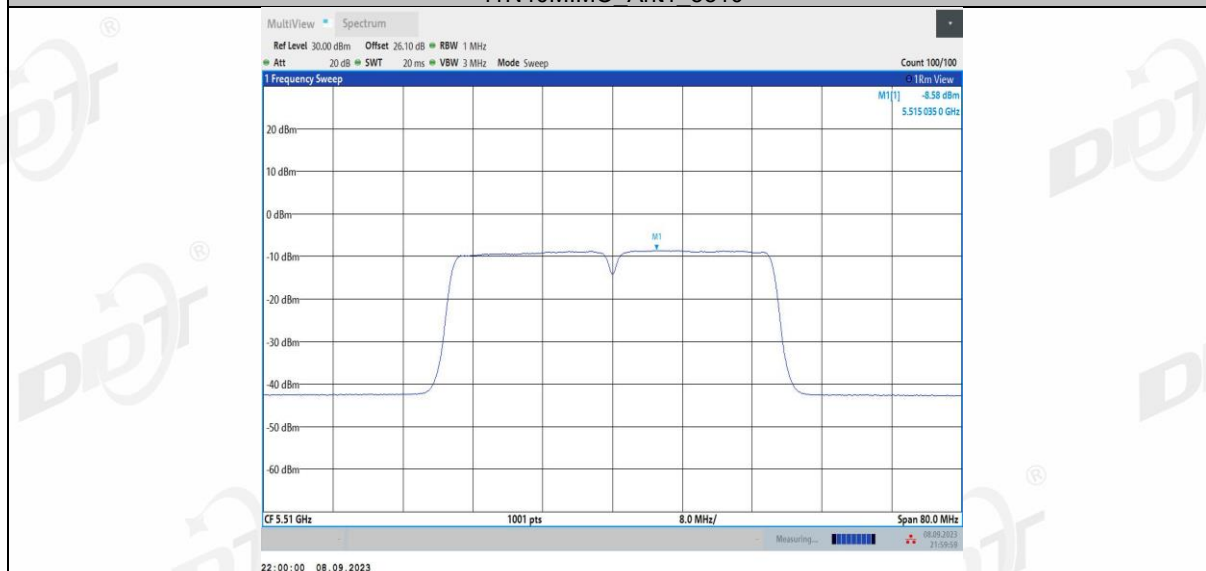
11N40MIMO_Ant2_5510
