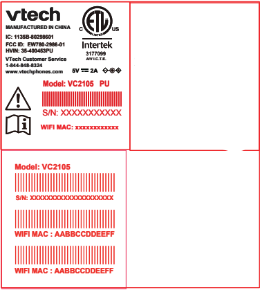
VC2105 PU LBL 50# PET SIZE: 56 x 62mm
