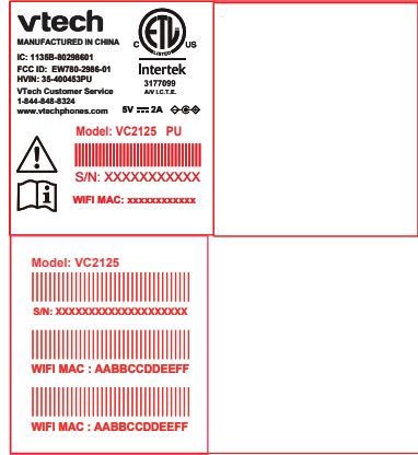
VC2125 PU LBL 50# PET SIZE: 56 x 62mm
