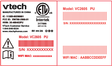
VC2605 PU LBL 50# PET SIZE: 55 x 32mm
