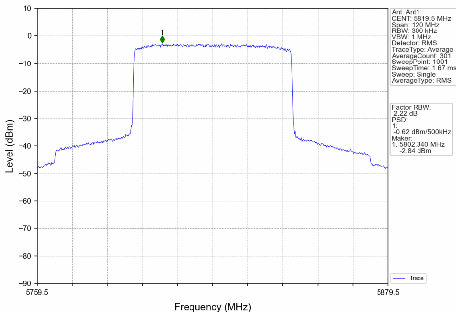
60MHz_HCH_5819.5MHz_Ant1_NTNV
