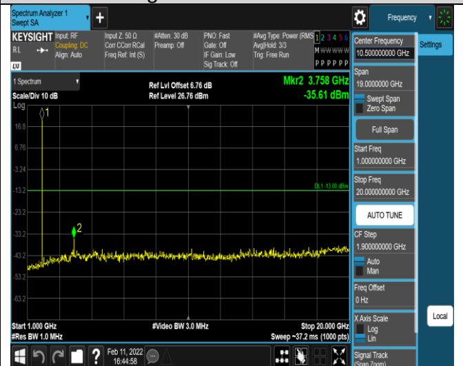
Band2-1.4MHz-QPSK-19193-1RB#0- Range2:1000~20000MHz
