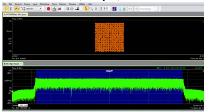
TM3.1a / 256QAM / 2655MHz
