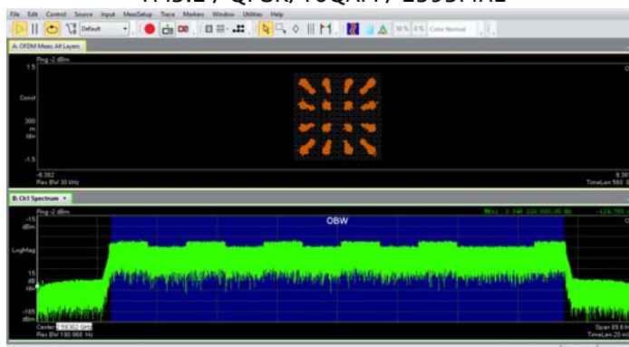
TM3.2 / QPSK/16QAM / 2593MHz
