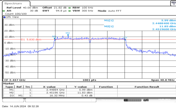
11G-CDD_Ant4_2457
