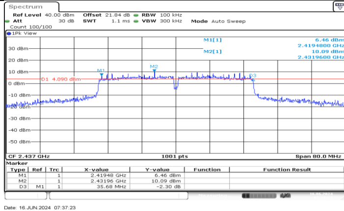
11N40MIMO_Ant4_2437
