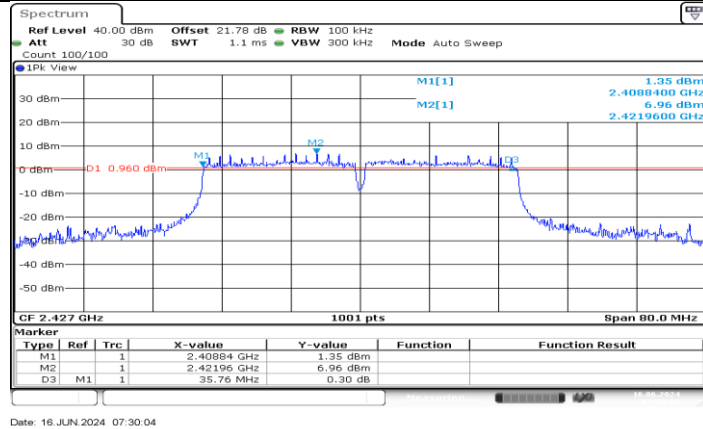
11N40MIMO_Ant3_2427
