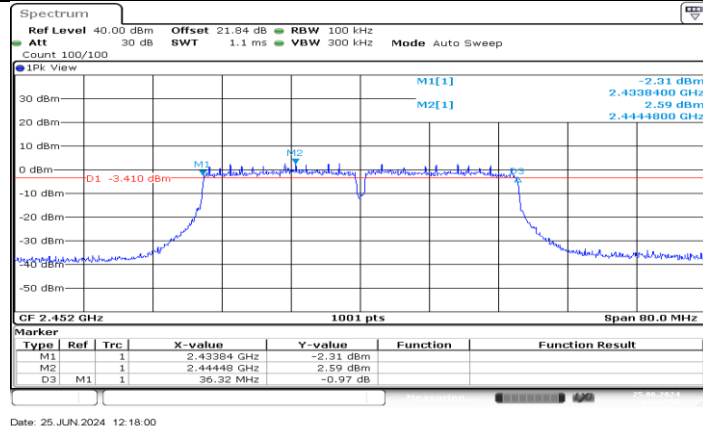
11N40MIMO_Ant3_2452
