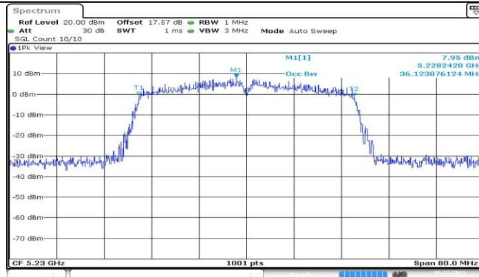
11N40MIMO_Ant1_5230
