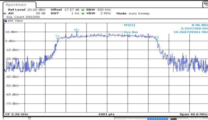
11AX20MIMO_Ant1_5260
