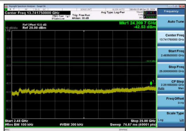
,Plot 4,2483.5MHz~25000MHz-802.11n(HT40),2452MHz,Ant0
