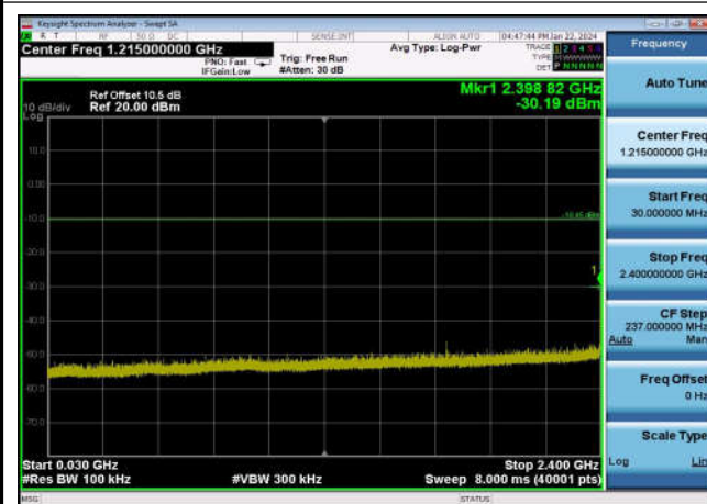
,Plot 3,30MHz~2400MHz-802.11b,2462MHz
