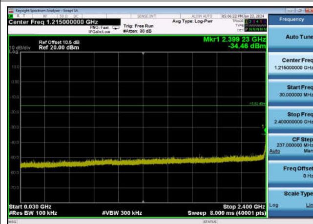
,Plot 3,30MHz~2400MHz-802.11g,2462MHz
