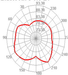
Bluetooth 0 TIS E1
