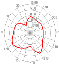
Bluetooth 19 TRP E1
