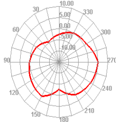
Bluetooth 0 TRP E2
