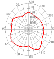
Bluetooth 39 TRP E1
